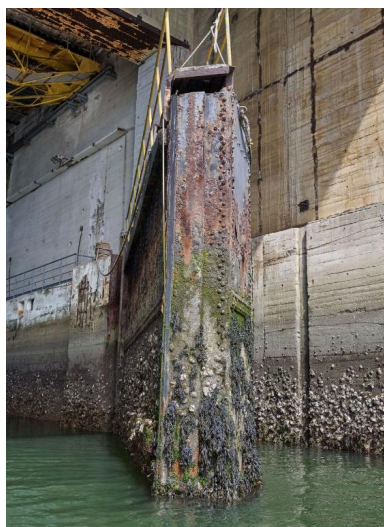
Vue de la porte est de l'alvéole G (n° 13 et 14) Phot. Bernard Bègne IVR53_20215600524NUCA
