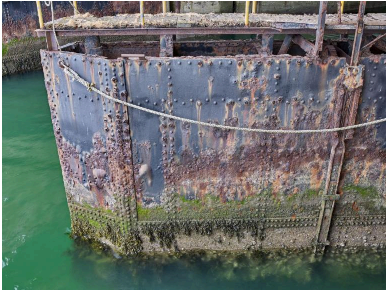
Vue de détail de la porte est de l'algéole G (n° 13 et 14)
