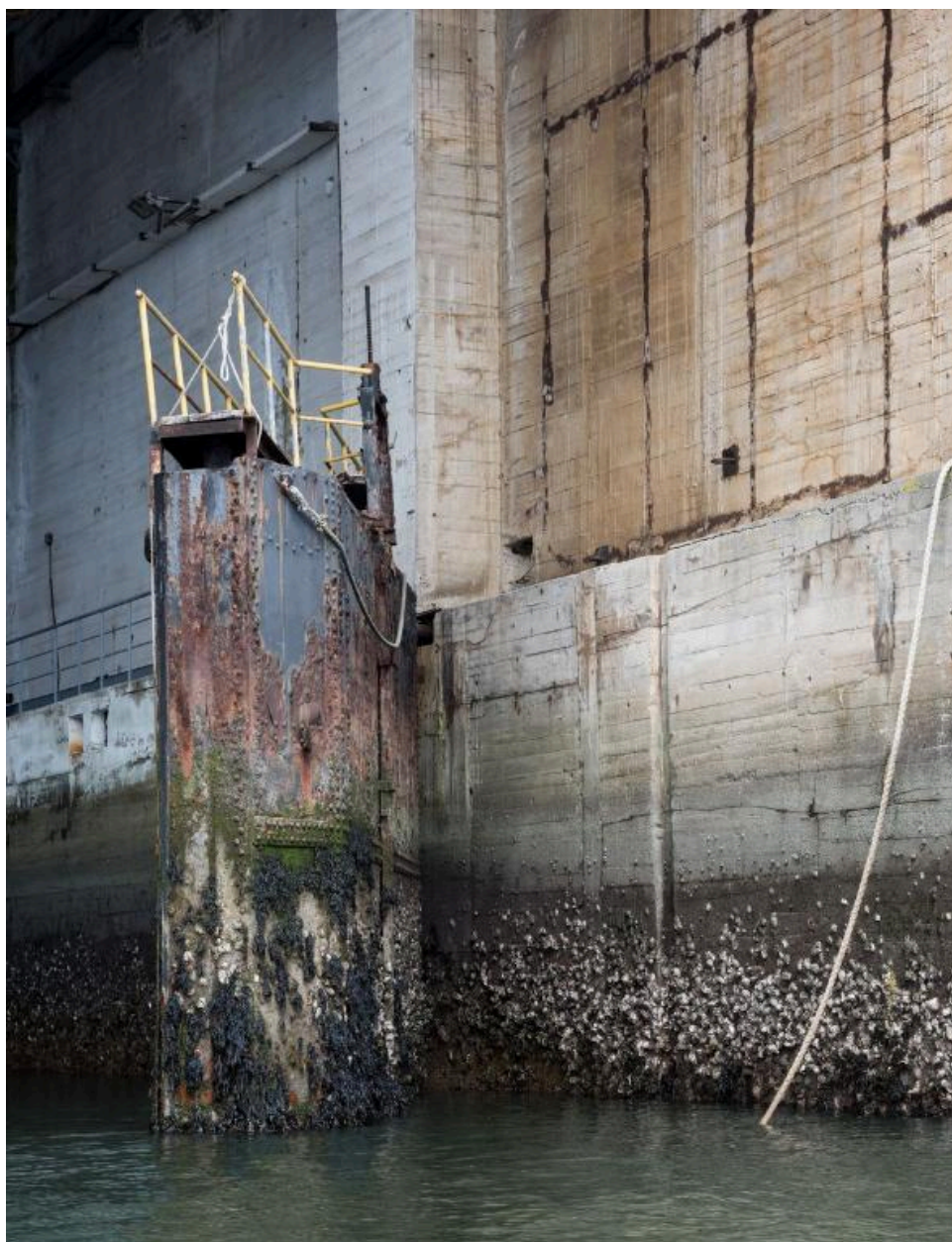
Vue de la porte est de l'algéole G (n° 13 et 14)
