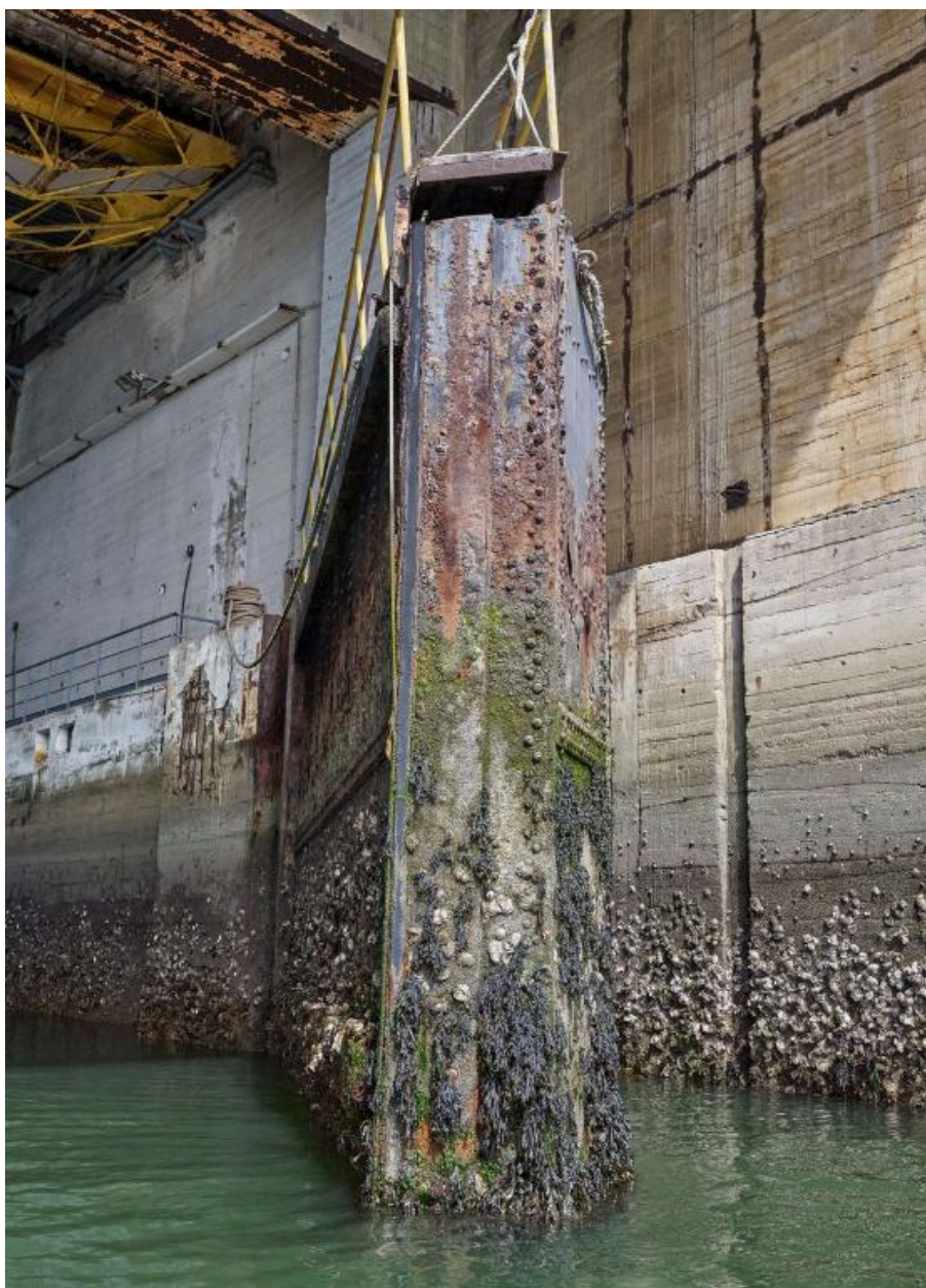
Vue de la porte est de l'algéole G (n° 13 et 14)
