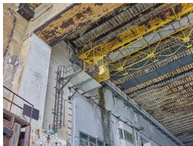
Vue de l'entrée de l'alvéole G (n° 13 et 14) : pont roulant d'une capacité de 5 tonnes Phot. Bernard Bègne IVR53_20215600525NUCA
