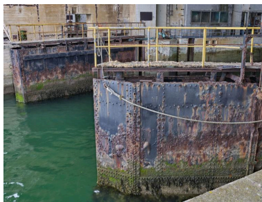
Vue des deux portes de l'alvéole G (n° 13 et 14) Phot. Bernard Bègne IVR53_20215600463NUCA
