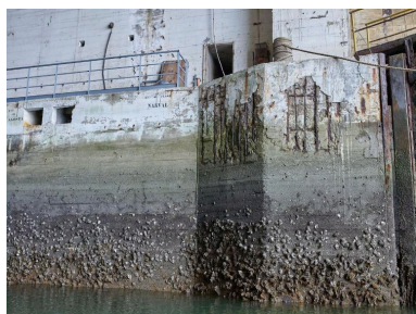
Vue de l'alvéole G (n° 13 et 14) : quai est n° 13, peintures murales françaises, repères d'amarrage pour les sous-marins de classe "AGOSTA" et "NARVAL"
