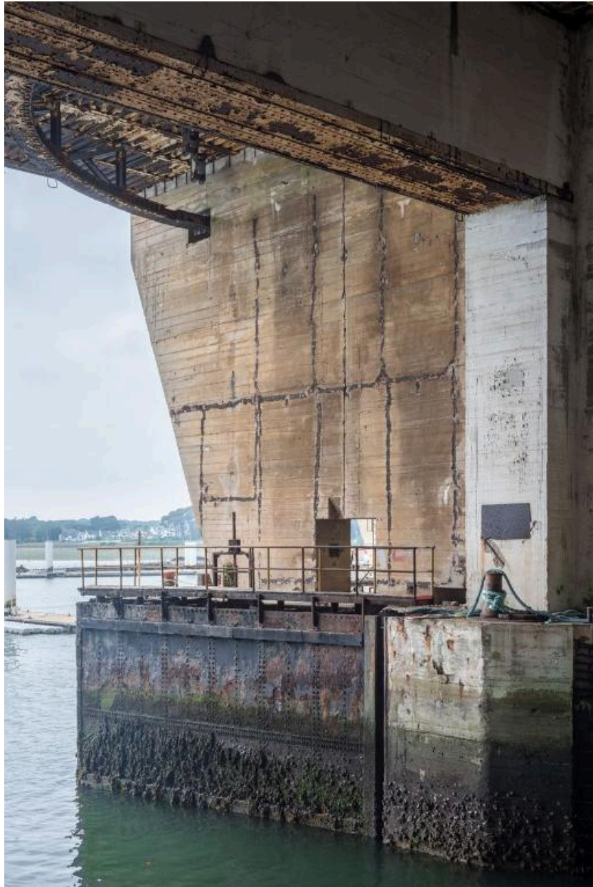
Vue de l'entrée de l'alcôve G (n° 13 et 14) : porte ouest et supports de fixation de la porte haute
