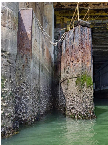
Vue de la porte ouest de l'alvéole G (n° 13 et 14)
