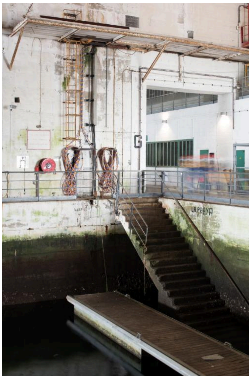
Vue de l'alvéole G (n° 13 et 14) : détail des équipements, escalier en béton armé
