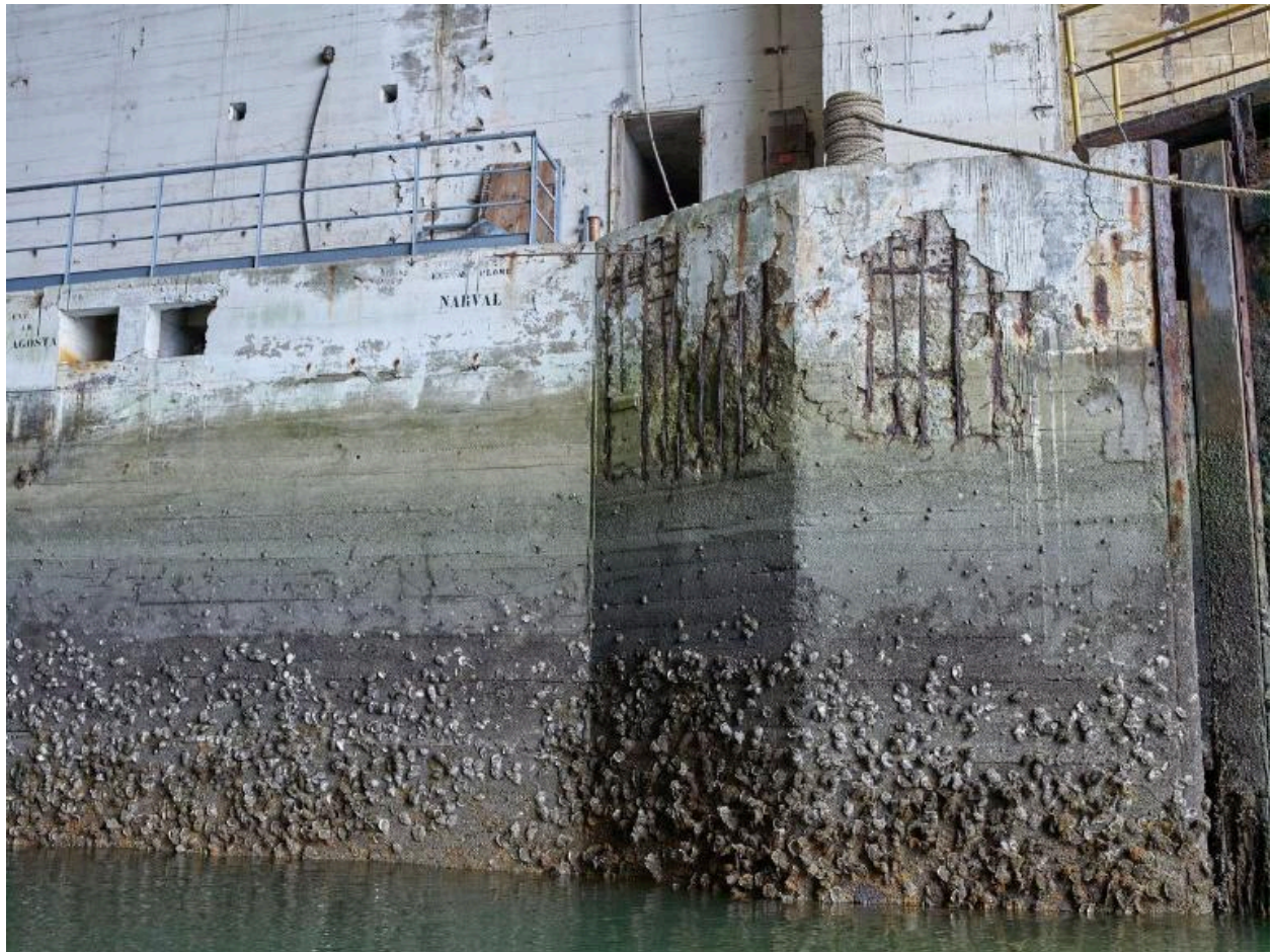
Vue de l'algéole G (n° 13 et 14) : quai est n° 13, peintures murales françaises, repères d'amarrage pour les sous-marins de classe "AGOSTA" et "NARVAL"
