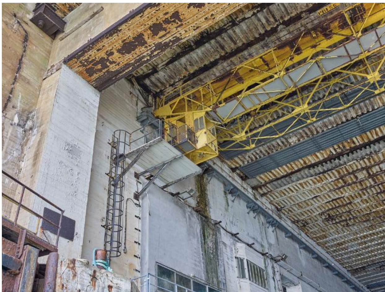
Vue de l'entrée de l'alcôve G (n° 13 et 14) : pont roulant d'une capacité de 5 tonnes
