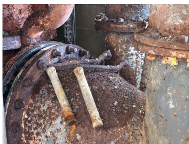
Vue de détail du corps/tuyau de pompe du bassin G. Deux manivelles sont posées sur le tuyau de pompe Phot. Bernard Bègne IVR53_20235600033NUCA
