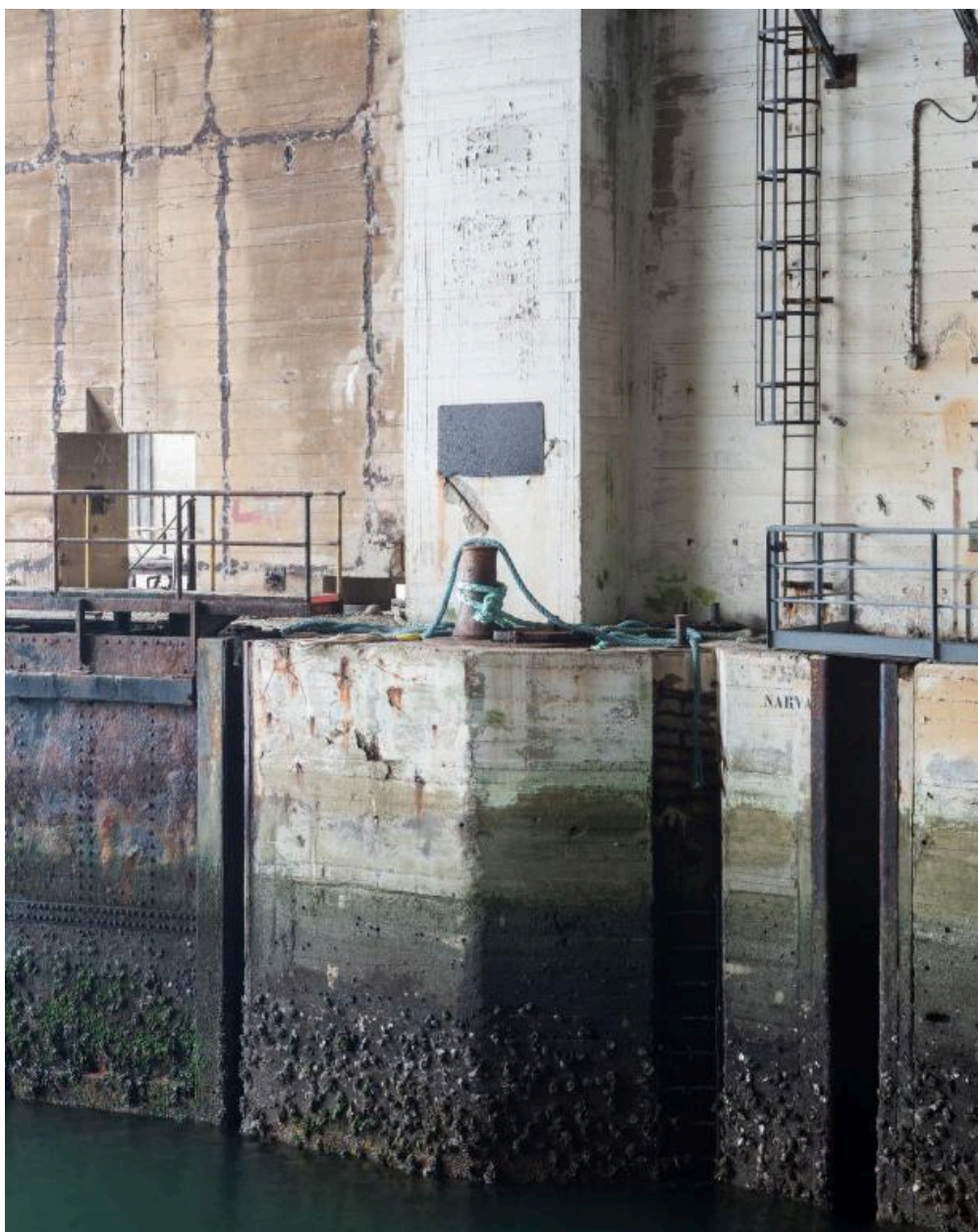
Vue de l'alvéole G (n° 13 et 14) : quai ouest n° 14, détail des équipements
