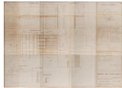
Plan d'installation des bouilleurs (plans et coupes), plan K n° 75, 5 juin 1946 (Service Historique de la Défense de Lorient, Monographie de la base "Ingénieur Général Stosskopf", 1945-1946) Phot. Service Historique de la Défense IVR53_20235605307NUCA
