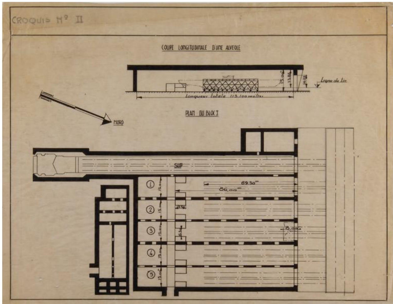
Plan et coupe longitudinale du bunker "K1", croquis II (Service Historique de la Défense de Lorient, Monographie de la base "Ingénieur Général Stoskopf", 1945-1946)
