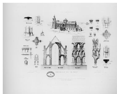
Elévations, coupes Repro. Guy Artur IVR53_19653500591Z
