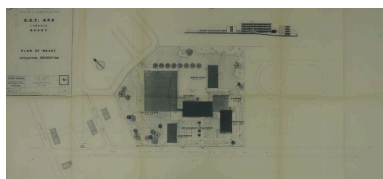
Plan masse du CET de Lanroze avec emplacement de la sculpture. Hervé Péron et Alexandre Weisbein, architectes (plan de 1973, modifié).
