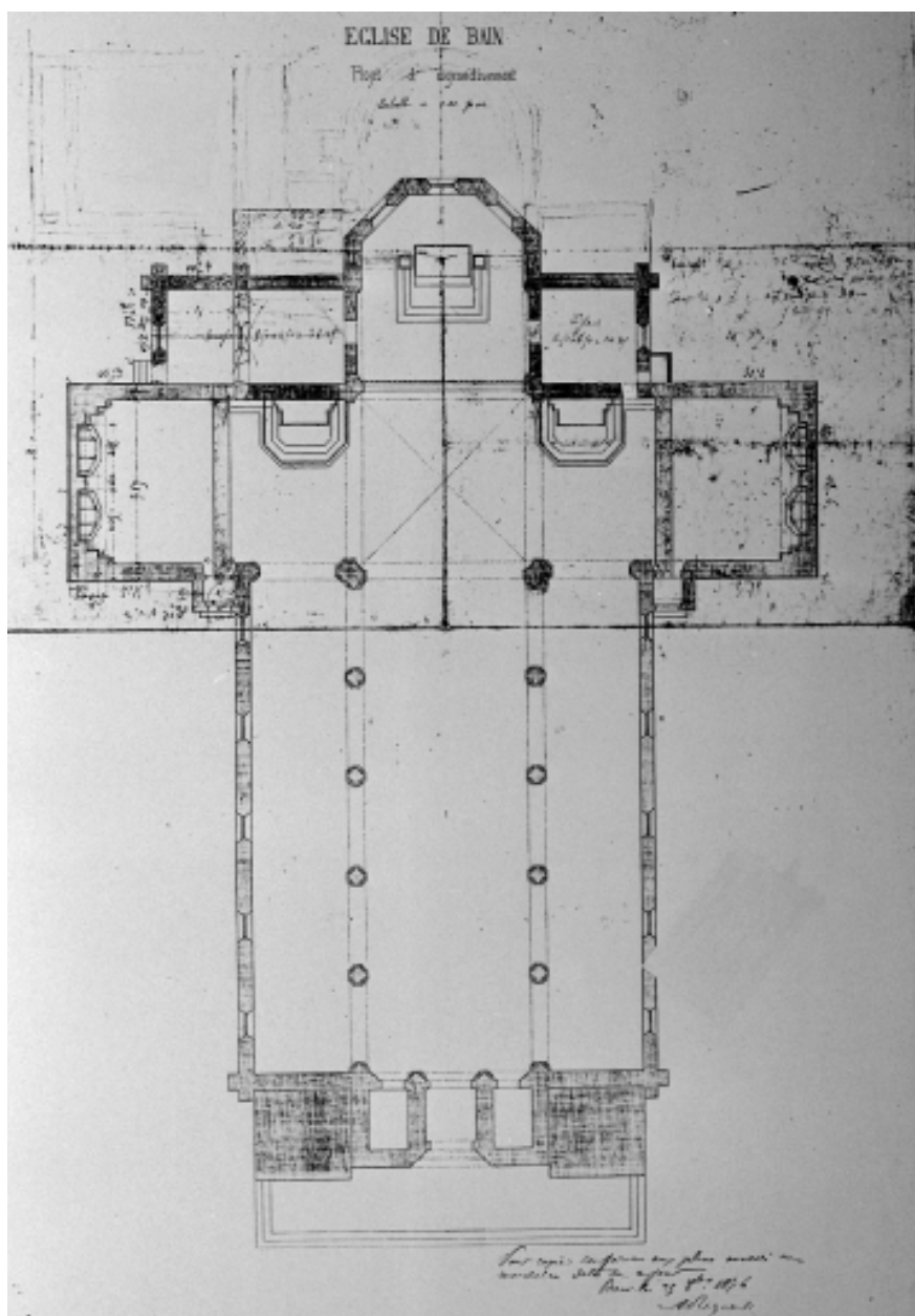
Plan au sol de l'église, projet d'agrandissement.
