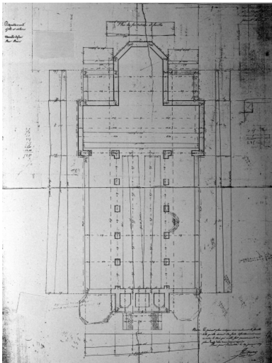
Plan des fondations et fouilles.
