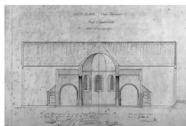
Coupe transversale, projet d'agrandissement. Phot. Auteur inconnu IVR53_19953500111V
