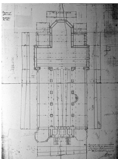
Plan des fondations et fouilles. Phot. Guy Artur, Phot. Norbert Lambart, Autr. Léonce Couëtoux IVR53_19973500202X
