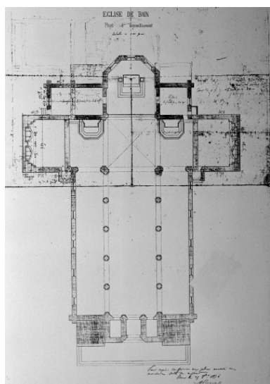
Plan au sol de l'église, projet d'agrandissement. Phot. Guy Artur, Phot. Norbert Lambart, Autr. Arthur Regnault IVR53_19973500203X
