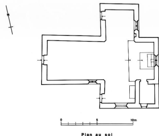
Plan au sol Phot. Guy Artur, Phot. Norbert Lambart, Phot. Auteur inconnu IVR53_19865600027P
