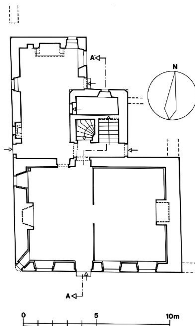
Plan au sol
