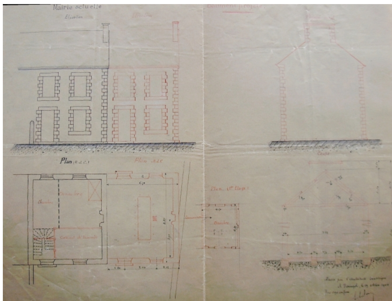
Ancienne école des garçons et mairie de Plounez, plan de l'architecte Hélyar, 19 octobre 1906 (AD 22)
