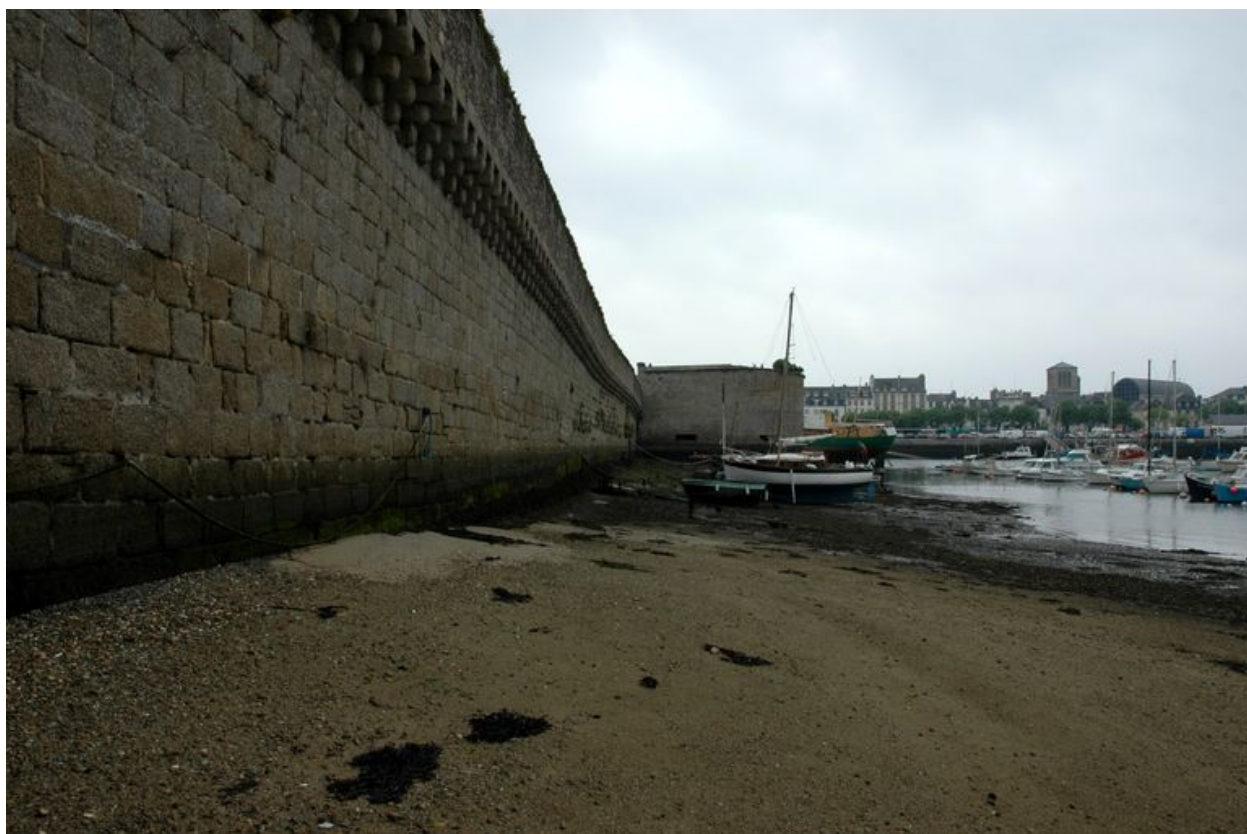
Vue de la ville-close de Concarneau : pied de la courtine située entre la tour de la Porte au Vin et la tour Neuve
