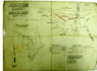
Plan du champ de mines Elorn I/192 (calque du service de déminage). Ce champ de mines composé de 571 mines antichar était implanté au nord du château de Roz ar Scour, entre le trait de côte et la route de la Corniche Phot. Guillaume Lécueillier IVR53_20022903095NUCA
