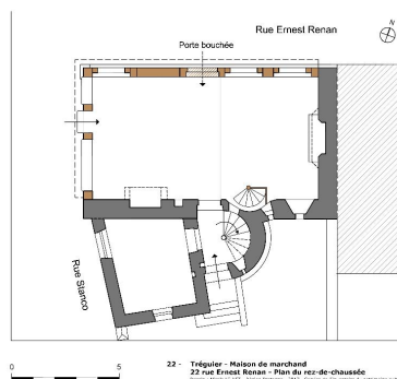
Plan au sol du rez-de-chaussée Dess. Nicole Le Net IVR53_20172202761NUDA
