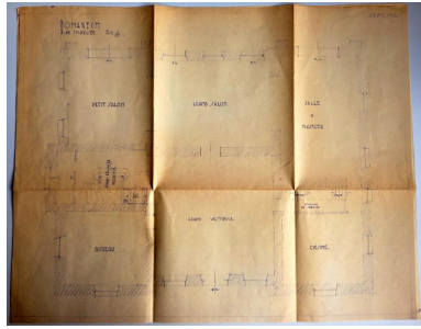
Plan de 1939 de la villa Rohannec'h : rez-de-chaussée Repro. Sophie Ehouarne IVR53_20262210039NUCA
