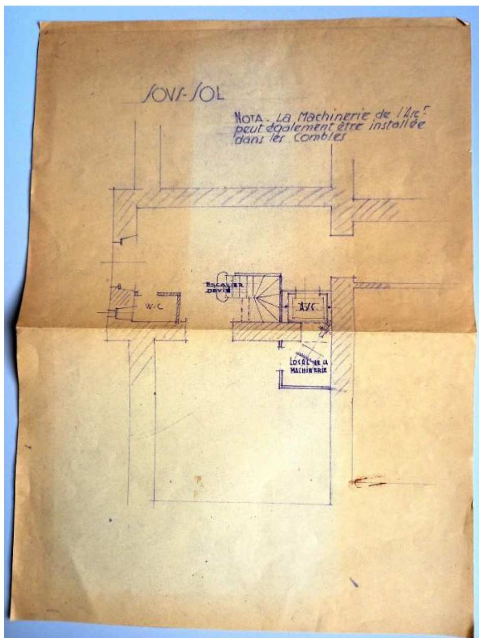
Plan de 1939 de la villa Rohannec'h : sous-sol
