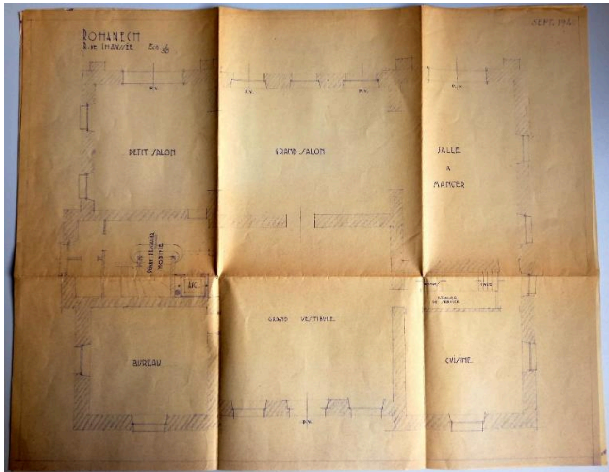
Plan de 1939 de la villa Rohannec'h : rez-de-chaussée
