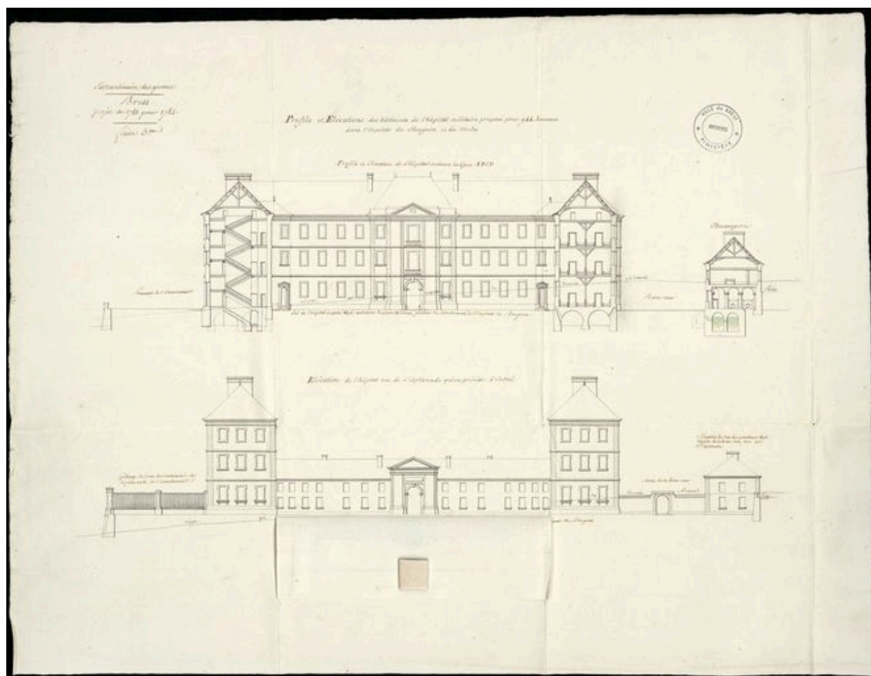
Projet d'hôpital militaire sur les hauteurs du Bouguen et du Menès à Brest, projet de 1781 pour 1782 : profils et élévations des bâtiments de l'hôpital militaire pour 944 hommes
