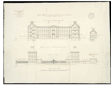
Projet d'hôpital militaire sur les hauteurs du Bouguen et du Menès à Brest, projet de 1781 pour 1782 : profils et élévations des bâtiments de l'hôpital militaire pour 944 hommes (entrée de l'hôpital) Phot. Archives municipales et communautaires. Brest Métropole Océane, Autr. Extraordinaire des Guerres IVR53_20082909079NUCA
