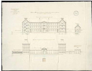
Projet d'hôpital militaire sur les hauteurs du Bouguen et du Menès à Brest, projet de 1781 pour 1782 : profils et élévations des bâtiments de l'hôpital militaire pour 944 hommes Phot. Archives municipales et communautaires. Brest Métropole Océane, Autr. Extraordinaire des Guerres IVR53_20082909080NUCA
