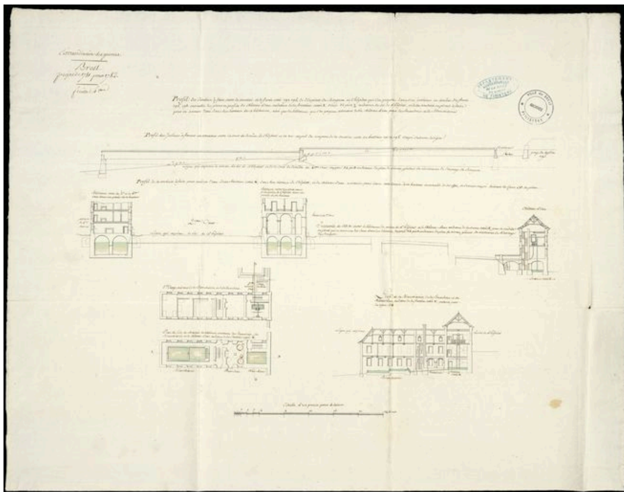
Projet d'hôpital militaire sur les hauteurs du Bouguen et du Menès à Brest, projet de 1781 pour 1782 : profils des jardins, du château d'eau au dessus de la fontaine, des citernes, de la buanderie et de la blanchisserie
