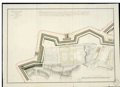
Projet d'hôpital militaire sur les hauteurs du Bouguen et du Menès à Brest, projet de 1781 pour 1782 : plan d'ensemble Phot. Archives municipales et communautaires. Brest Métropole Océane, Autr. Extraordinaire des Guerres IVR53_20082909074NUCA
