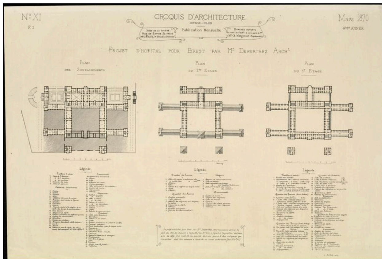
Projet d'hôpital pour Brest par Edouard Deperthes, architecte de la ville de Brest : plan général et légende, Intime-club, croquis d'architecture, publication mensuelle, mars 1870
