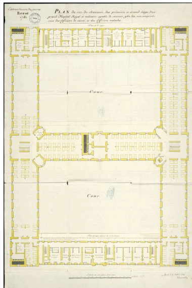
Projet d'hôpital militaire à Brest, projet de 1781, fait à Brest le 4 juillet 1781 par Dumoulin : plan d'un grand hôpital Royal et militaire capable de contenir 960 lits, plan du 1er étage Phot. Archives municipales et communautaires. Brest Métropole Océane, Autr. Dumoulin IVR53_20082909083NUCA
