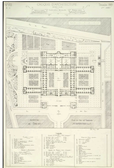
Projet d'hôpital pour Brest par Edouard Deperthes, architecte de la ville de Brest : plan général et légende, Intime-club, croquis d'architecture, publication mensuelle, décembre 1869 Phot. Archives municipales et communautaires. Brest Métropole Océane, Autr. Edouard Deperthes IVR53_20082909092NUCA
