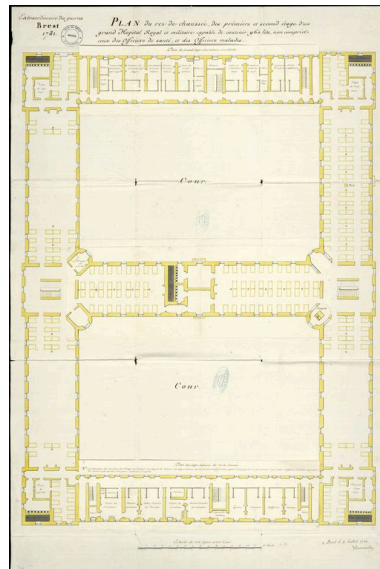
Projet d'hôpital militaire à Brest, projet de 1781, fait à Brest le 4 juillet 1781 par Dumoulin : plan d'un grand hôpital Royal et militaire capable de contenir 960 lits, plan du 2ème étage Phot. Archives municipales et communautaires. Brest Métropole Océane, Autr. Dumoulin IVR53_20082909082NUCA
