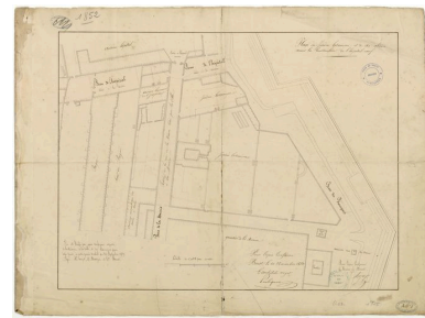
Quartier de l'Harteloire : plan du jardin botanique de Brest et de ses abords avant la construction de l'hôpital neuf, 1839 (expertise), 1852 (copie conforme par Pouliquen, signature du maire de Brest). Nouvelles constructions en surimpression. Phot. Archives municipales et communautaires. Brest Métropole Océane, Autr. architecte. Auguste Pouliquen Voyer IVR53_20082909090NUCA
