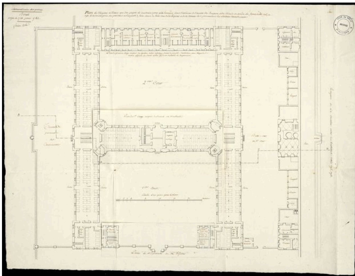
Projet d'hôpital militaire sur les hauteurs du Bouguen et du Menès à Brest, projet de 1781 pour 1782 : plan général de l'hôpital militaire pour 944 hommes, de la boulangerie, des pavillons et hangars de la basse cour et de la terrasse
