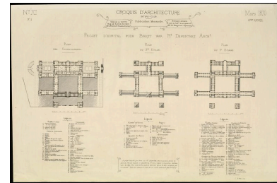
Projet d'hôpital pour Brest par Edouard Deperthes, architecte de la ville de Brest : plan général et légende, Intime-club, croquis d'architecture, publication mensuelle, mars 1870 Phot. Archives municipales et communautaires. Brest Métropole Océane, Autr. Edouard Deperthes IVR53_20082909093NUCA
