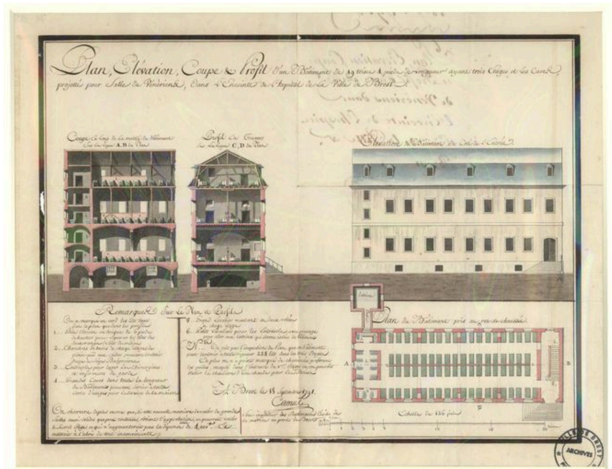
Plan, élévation, coupe et profil d'un bâtiment de 19 toises 4 pieds de longueur ayant trois étages et les caves projeté pour salle de vénériens dans l'enceinte de l'hôpital de la ville de Brest, fait à Brest le 18 septembre 1791 par Camus
