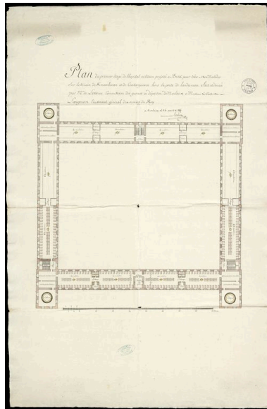
Plan du 1er étage d'un hôpital militaire pour 1500 à 1800 malades sur le terrain de Keranbecan et de Coatargueven hors de la porte de Landerneau à Brest, fait à Morlaix le 15 août 1786 par Lasserre adressé à Langeron, lieutenant général Phot. Archives municipales et communautaires. Brest Métropole Océane, Autr. ? de Lasserre IVR53_20082909085NUCA
