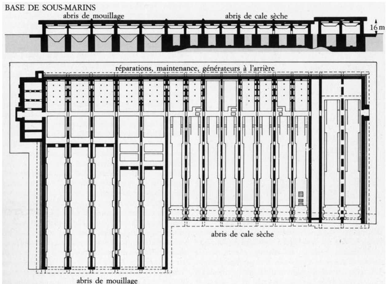
Plan et coupe de la base de sous-marins de Brest (planche publiée en 1983)
