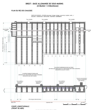
Plan, coupe et chronologie de la base de sous-marins de Brest (planche publiée en 2011) Phot. Guillaume Lécueillier, Phot. Nicole Le Net IVR53_20222905841NUCA
