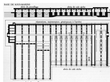
Plan et coupe de la base de sous-marins de Brest (planche publiée en 1983) Repro. Guillaume Lécuyer IVR53_20042904065NUCA
