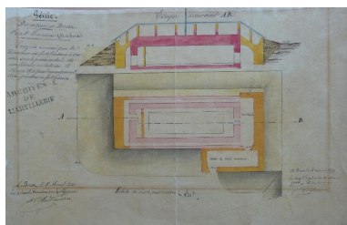
3 W 58. Croquis annexé par le Directeur des fortifications à son avis sur le procès-verbal de conférence en date du 18 mars 1870, pour l'emmagasinement des poudres au fort Lacroix, 5 avril 1870. Phot. Patrick Jadé IVR53_20175606845NUCA
