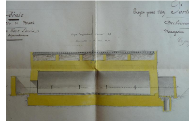
1 VH 1474. Place de Port-Louis, feuille n° 4 des projets pour 1849, achèvement du fort Lacroix, magasin à poudre pour 30000 kg, 17 décembre 1848. Phot. Patrick Jadé IVR53_20175606841NUCA
