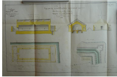
1 VH 1474. Place de Port-Louis, feuille n° 4 des projets pour 1849, achèvement du fort Lacroix, magasin à poudre pour 30000 kg, 17 décembre 1848. Phot. Patrick Jadé IVR53_20175606840NUCA
