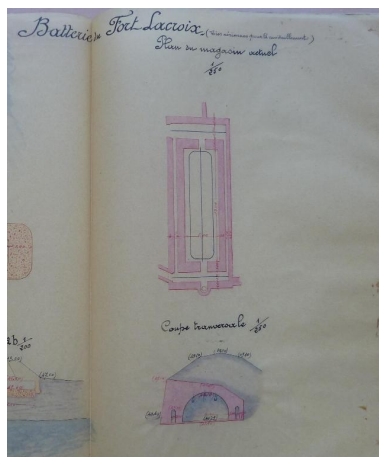
7 N 1905. Croquis joint au procès-verbal de conférence du 15 novembre 1894, emmagasinement des munitions dans la place de Lorient-Groix, fort Lacroix. Phot. Patrick Jadé IVR53_20175606846NUCA
