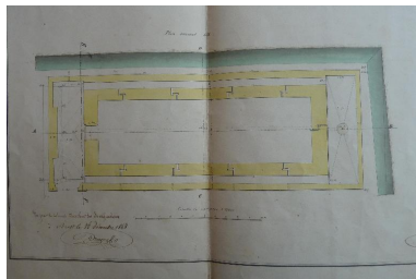
1 VH 1474. Place de Port-Louis, feuille n° 4 des projets pour 1849, achèvement du fort Lacroix, magasin à poudre pour 30000 kg, 17 décembre 1848. Phot. Patrick Jadé IVR53_20175606842NUCA
