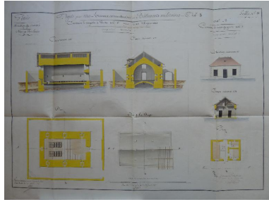
1 VH 1473. Place de Port-Louis, feuille n° 11 des projets extraordinaires pour 1845, construire le magasin à poudre coté C pour 20000 kilogrammes, 28 décembre 1845. Phot. Patrick Jadé IVR53_20175606839NUCA
