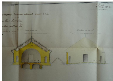
1 VH 1474. Place de Port-Louis, feuille n° 4 des projets pour 1849, achèvement du fort Lacroix, magasin à poudre pour 30000 kg, 17 décembre 1848. Phot. Patrick Jadé IVR53_20175606843NUCA
