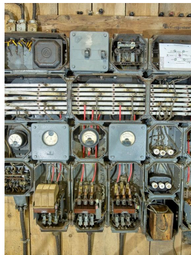
Vue intérieure : salle des machines pour deux groupes électrogènes, détail du tableau électrique de la batterie antiaérienne Rossitten Phot. Bernard Bègne IVR53_20255600881NUCA
