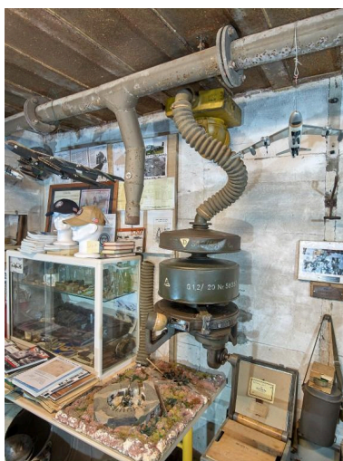
Vue intérieure : atelier, système de ventilation et de filtration avec ventilateur de 1,2 m3, filtre dépoussiéreur et tuyauterie d'origine en place (les filtres sont rapportés). Ce bunker-musée a pour thématique la Seconde Guerre mondiale Phot. Bernard Bègne IVR53_20255600893NUCA
