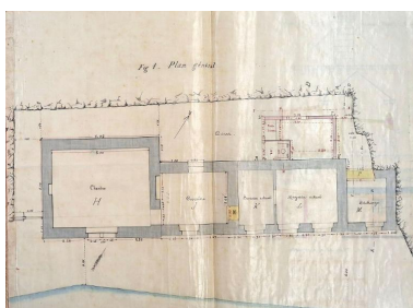
Plan général des modifications à apporter aux logement du gardien de phare, bureau et magasin aux huiles des Ponts-et-Chaussées (1894) Repro. Erwana L'Haridon IVR53_20262210090NUCA
