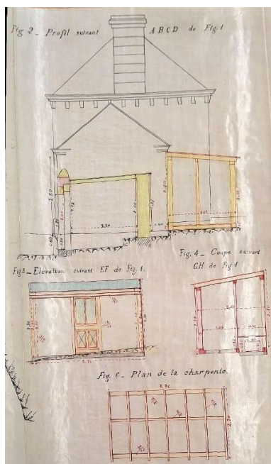
Plan des modifications : profil et élévation du bureau et du magasin aux huiles des Ponts-et-Chaussées (1894) Repro. Erwana L'Haridon IVR53_20262210091NUCA
