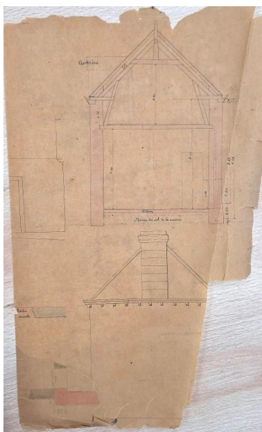
Plan des modifications à apporter : coupe de l'ancien bureau et magasin aux huiles des Ponts-et-Chaussées (1887) Repro. Erwana L'Haridon IVR53_20262210093NUCA
