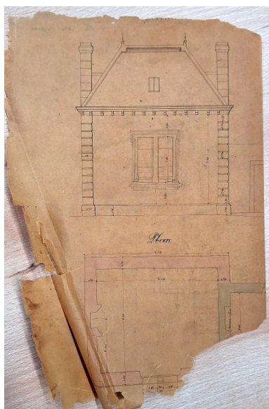
Plan des modifications à apporter : élévation du bureau et du magasin aux huiles des Ponts-et-Chaussées (1887) Repro. Erwana L'Haridon IVR53_20262210092NUCA
