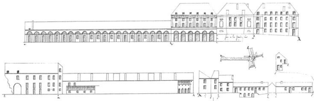
Elévations des établissements maritimes du port de Brest, année 1807. Magasin Général (face à la grande rue). Plan d'ensemble
