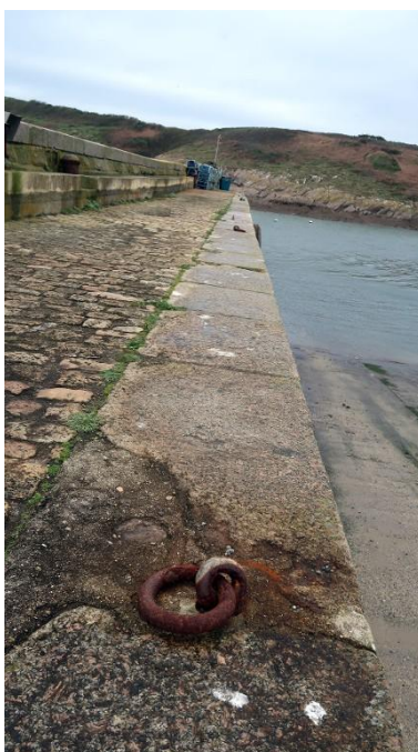
Môle Saint-Christophe : pierre de taille, pavés et anneaux d'amarrage Phot. Erwana L'Haridon IVR53_20242910180NUCA
