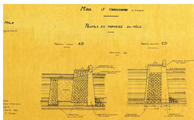
Profils de travers du môle Saint-Christophe, ingénieur A. Cahen, février 1870 IVR53_20232905848NUCA
