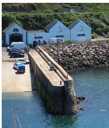
Môle Saint-Christophe, vue du couronnement et de la mise en œuvre des maçonneries Phot. Erwana L'Haridon
