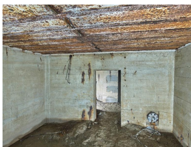
Vue du magasin à munitions situé au sud. Sur le mur du fond : câblage électrique pour l'alimentation des plafonniers et à droite, bouche de surpression à clapet à contrepoids
