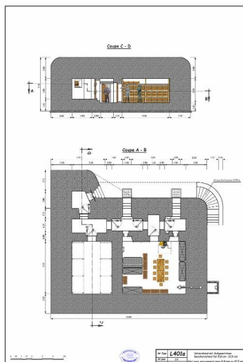
Plan et coupe d'un bunker-abri-magasin de munitions de type L 401a avec cuve pour canon antiaérien de 10,5 cm (Unterstand mit aufgesetztem Geschützstand für 8,8/10,5 cm Flak) Dess. Christian Moigne IVR53_20263510107NUDA
