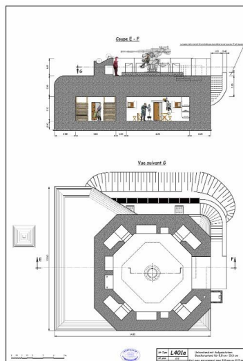
Plans et coupes d'un bunker-abri-magasin de munitions de type L 401a avec cuve pour canon antiaérien de 10,5 cm (Unterstand mit aufgesetztem Geschützstand für 8,8/10,5 cm Flak) Dess. Christian Moigne IVR53_20263510108NUDA
