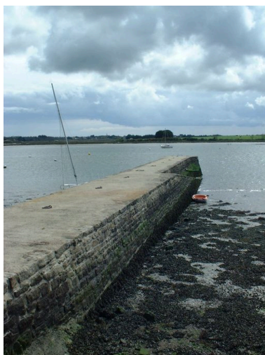
Vue générale de la jetée de la Garenne Phot. Julien Amghar IVR53_20085606106NUCA
