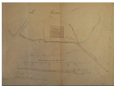
Plan ancien de la jetée de la Garenne datant de 1853 Phot. Julien Amghar, Phot. Auteur inconnu, Autr. Auteur inconnu IVR53_20085606111NUC
