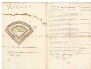
Profil et plan type d'une batterie de mortier du Goulet de Brest avec un état des batteries de mortier qui défendent cette rade, fait à Brest le 2 janvier 1693 par Champy Desclouzeaux, intendant de Brest de 1683-1701 Repr. Service historique de la Défense, Autr. Champy Desclouzeaux IVR53_20082908860NUCA
