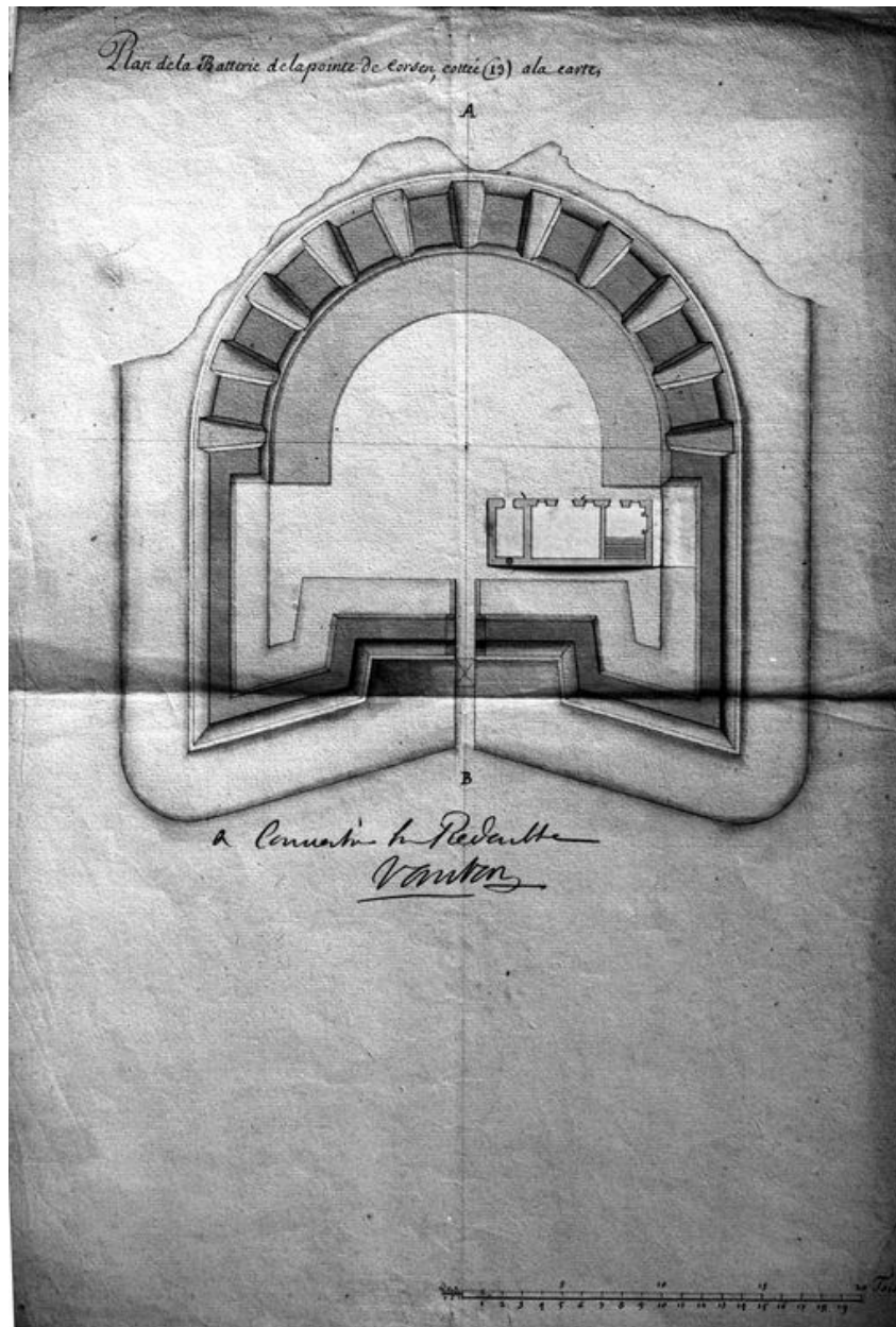
Plan de la batterie de la pointe de Corsen (projet : ?, commune de Plouarzel) par Vauban
