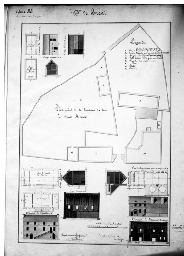
Atlas des bâtiments militaires des places de France : direction de Brest, arrondissement du Conquet : plan général de la manutention des vivres à Saint-Renan, vers 1836 Repro. Guy Artur, Repro. Norbert Lambart, Autr. IVR53_19862902795NUC
