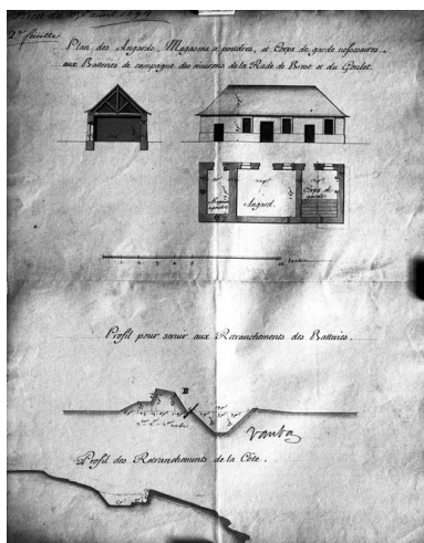
Plan des hangars, magasins à poudre et corps de garde nécessaires aux batteries de campagne des environs de la rade de Brest et du Goulet, avril 1694 Repro. Guy Artur, Repro. Norbert Lambart IVR53_19832900732PB
