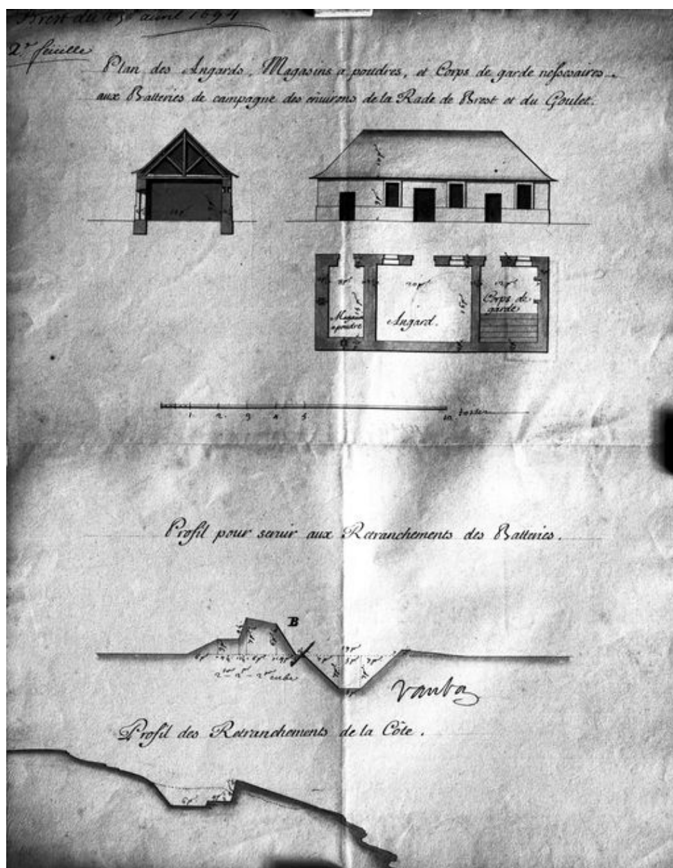
Plan des hangars, magasins à poudre et corps de garde nécessaires aux batteries de campagne des environs de la rade de Brest et du Goulet, avril 1694
