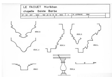
Plan, détail : a,b,c,d,e,f,g. Relevés des moulurations des fenêtres et des portes. Phot. Auteur inconnu IVR53_19775600179V
