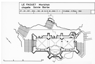
Plan au sol. Phot. Auteur inconnu, Autr. G. Lefranc, Autr. G. Peron IVR53_19775600196V
