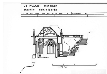
Coupe transversale sur l'abside, V-V (1965). Phot. Auteur inconnu, Autr. G Lefranc IVR53_19775600207V
