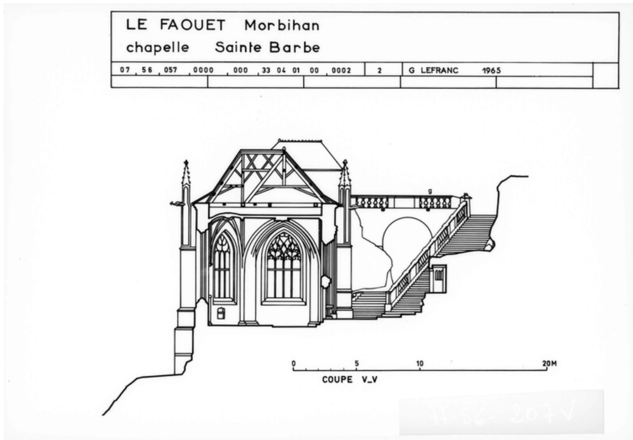
Coupe transversale sur l'abside, V-V (1965).
