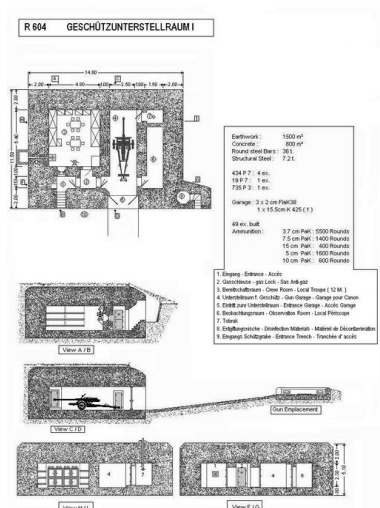
Plan d'un bunker - casemate de type 604 (dessin : Patrick Fleuridas) Phot. Patrick Fleuridas IVR53_20042904369NUCA
