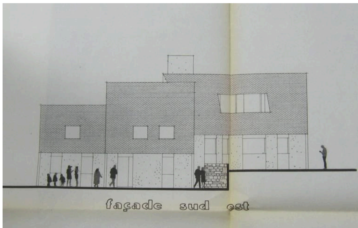
Façade Sud-Est, P. Talou, L. Bizouarn
