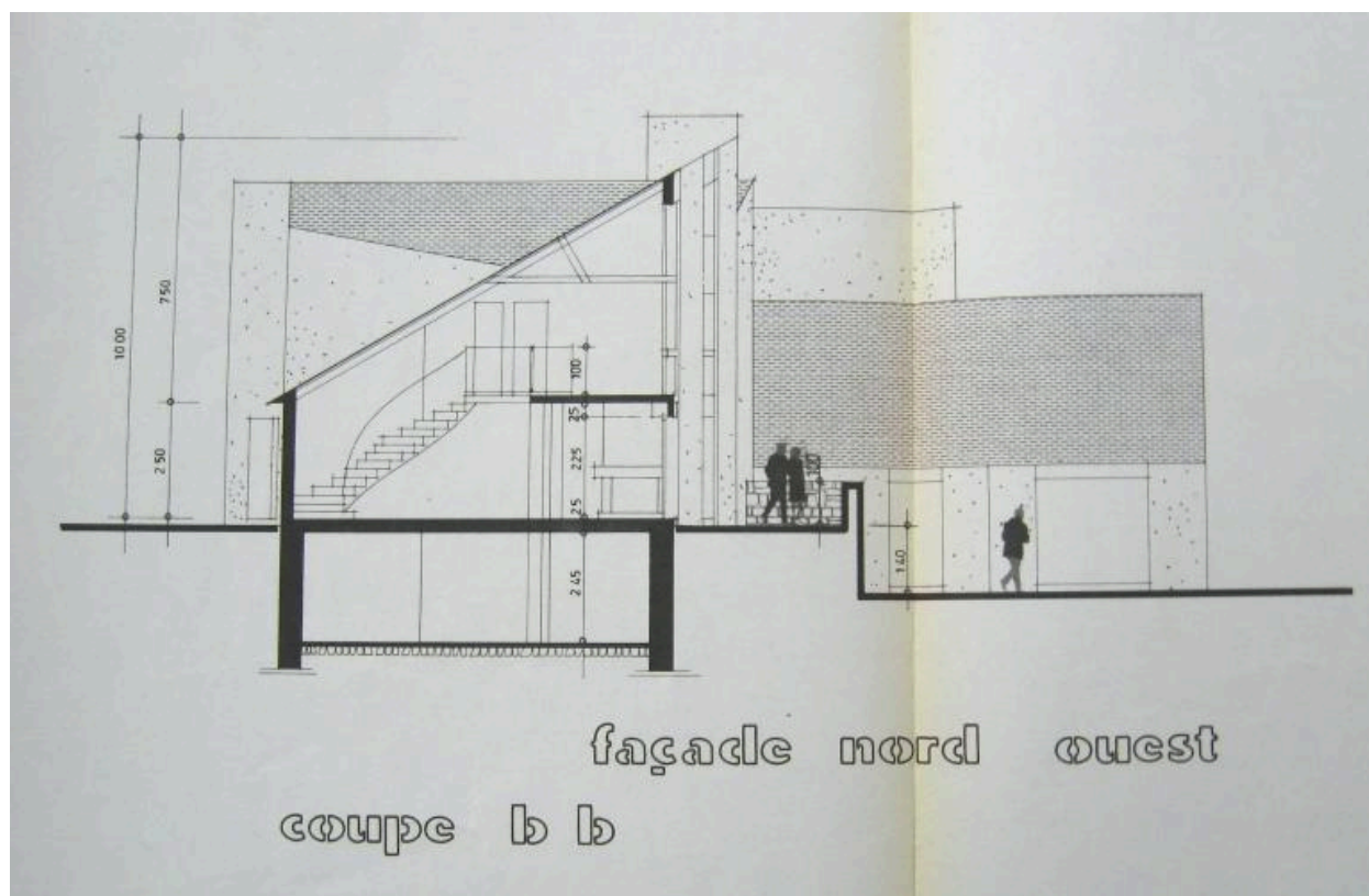
Coupe Façade Nord-Ouest, L. Bizouarn - P. Talou
