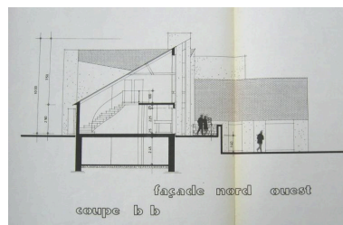
Coupe Façade Nord-Ouest, L. Bizouarn - P. Talou Dess. Pierre Talou, Dess. Louis Bizouarn IVR53_20225605076A0
