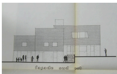
Façade Sud-Est, P. Talou, L. Bizouarn Dess. Pierre Talou, Dess. Louis Bizouarn IVR53_20225605077A0
