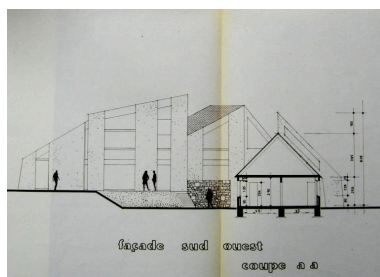
Coupe Façade Sud-Ouest, L. Bizouarn, P. Talou Dess. Pierre Talou, Dess. Louis Bizouarn IVR53_20225605078A0
