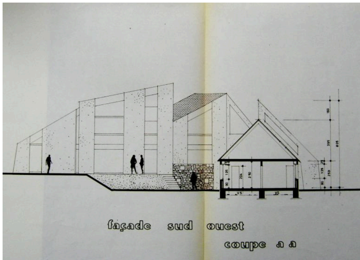
Coupe Façade Sud-Ouest, L. Bizouarn, P. Talou
