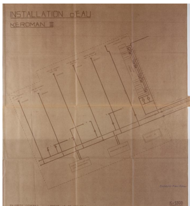
Plan du circuit d'installation d'eau douce du bunker "KIII" (eau potable et incendie), plan K n
