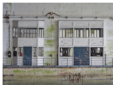
Vue générale de la salle des pompes de l'alvéole D (quai n° 19) aménagée dans l'épaisseur du mur de refend Phot. Bernard Bègne IVR53_20235600110NUCA
