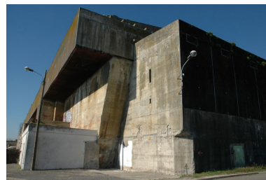
Vue de l'angle nord-est : gigantisme du contrefort et de la dalle de couverture en béton armé (2005) Phot. Guillaume Lécueillier IVR53_20055603568NUCA
