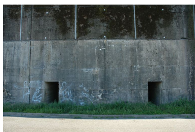
Vue de deux entrées protégées, aménagées dans l'élévation nord, front arrière (2005) Phot. Guillaume Lécueillier IVR53_20055603577NUCA
