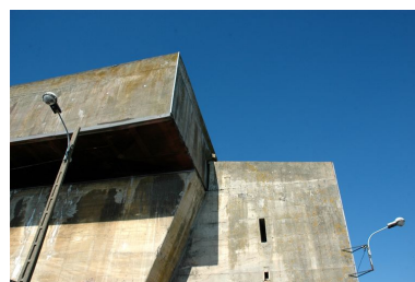
Vue de l'angle nord-est : gigantisme du contrefort et de la dalle de couverture en béton armé (2005) Phot. Guillaume Lécueillier IVR53_20055603575NUCA
