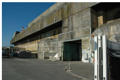
Vue de l'entrée est flanquée de deux casemates pour mitrailleuse et surmontée d'un observatoire (2005) Phot. Guillaume Lécueillier IVR53_20055603566NUCA
