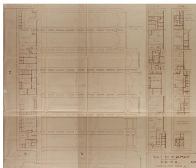
Plan d'ensemble du bunker "KIII" : bassins et locaux, plan K n ° 5, 11 décembre 1945 (Service Historique de la Défense de Lorient, Monographie de la base "Ingénieur Général Stosskopf", 1945-1946)
