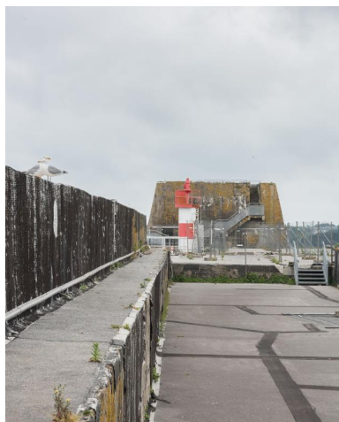
Vue de l'un des bunkers destinés à la défense antiaérienne regroupant encuvement et abri pour les soldats. Au premier plan à gauche, poutres longitudinales des chambres d'explosion (inachevées). A signaler : dispositif de signalisation maritime babord
