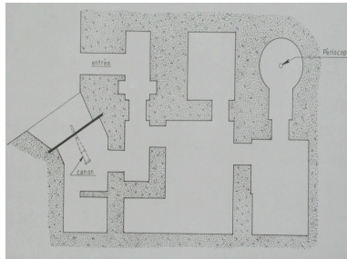
Plan type du blockhaus de Château-Tanguy, par Michel Piéto (collection particulière) Repro. Guy Prigent, Autr. Michel Piéto IVR53_20032205091NUCB
