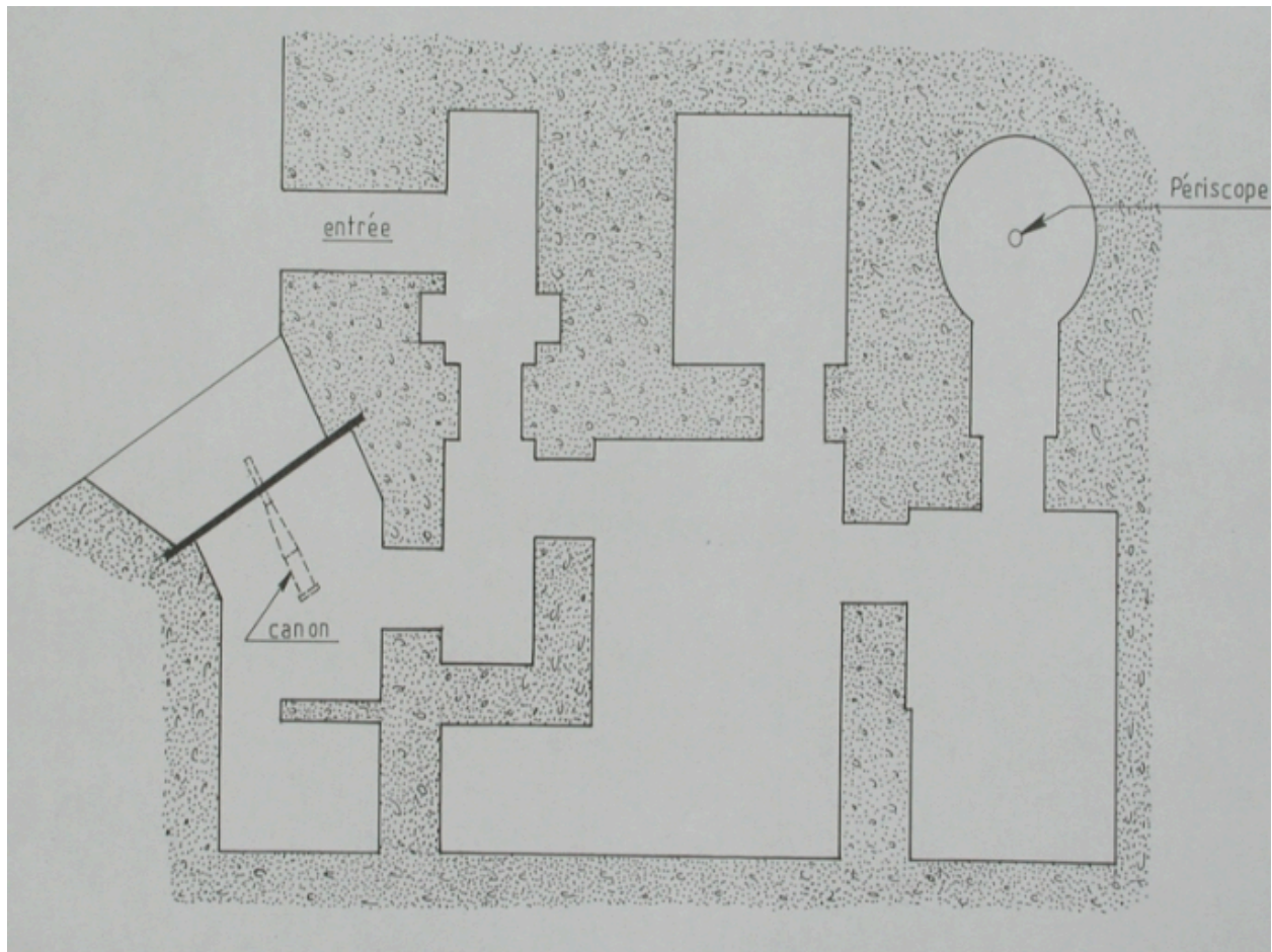
Plan type du blockhaus de Château-Tanguy, par Michel Piéto (collection particulière)
