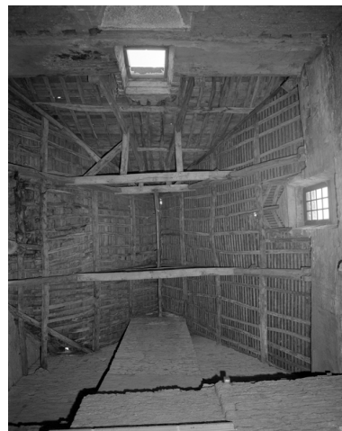
Charpente
