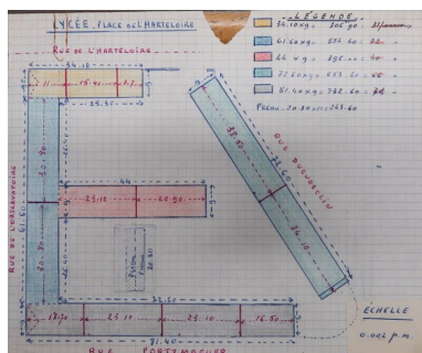
Plan du lycée en baraques. Sans nom ni date (vers 1945). Autr. Auteur inconnu (document reproduit) IVR53_20242911456A1
