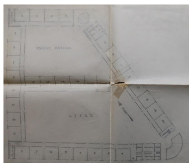
Plan du lycée et du collège moderne en baraques (implantation provisoire pour ce dernier, d'octobre 1945 à juillet 1946). Sans nom ni date. Autr. Auteur inconnu (document reproduit) IVR53_20242911459A1
