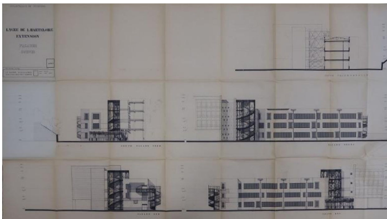
Extension : Elévations. Jean-Paul Huéber, architecte, 1988.
