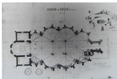
Plan d'ensemble de l'église et extrait du plan cadastral, 1891 Repro. Norbert Lambert IVR53_19973504802X
