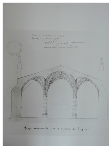
Coupe transversale sur le milieu de l'église, 1891 Repro. Norbert Lambert IVR53_19973504803X
