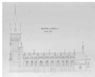
Plan de la façade sud Repro. Norbert Lambert IVR53_19973500092X
