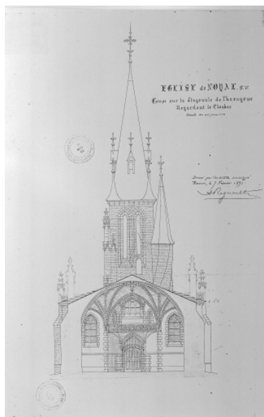
Plan de la façade ouest Repro. Norbert Lambert IVR53_19973500283X
