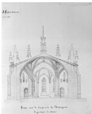
Coupe sur la diagonale de l'hexagone Phot. Norbert Lambert IVR53_19973500284X
