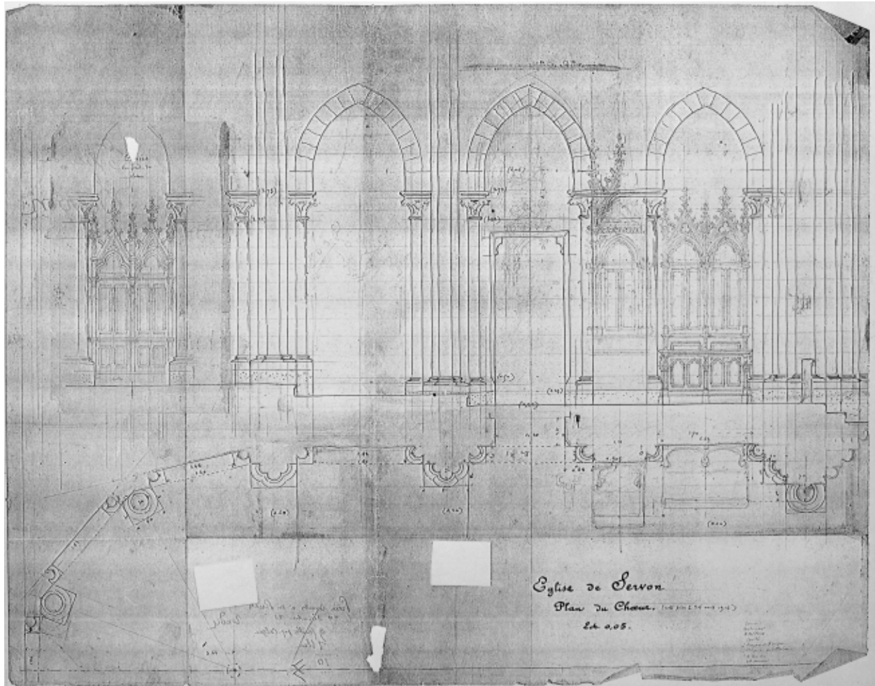
Plan du chœur, 1914, attribué à A. Regnault
