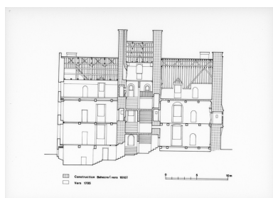
Coupe avec époques de construction Phot. Guy Artur, Phot. Norbert Lambart IVR53_19892200003P
