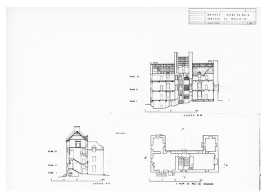
Plan et coupes Phot. François Dagorn IVR53_19762200089P
