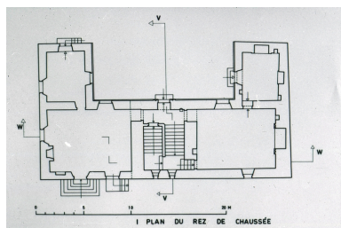
Plan du rez-de-chaussée Phot. Guy Artur, Autr. P Boutroux IVR53_19762200375P
