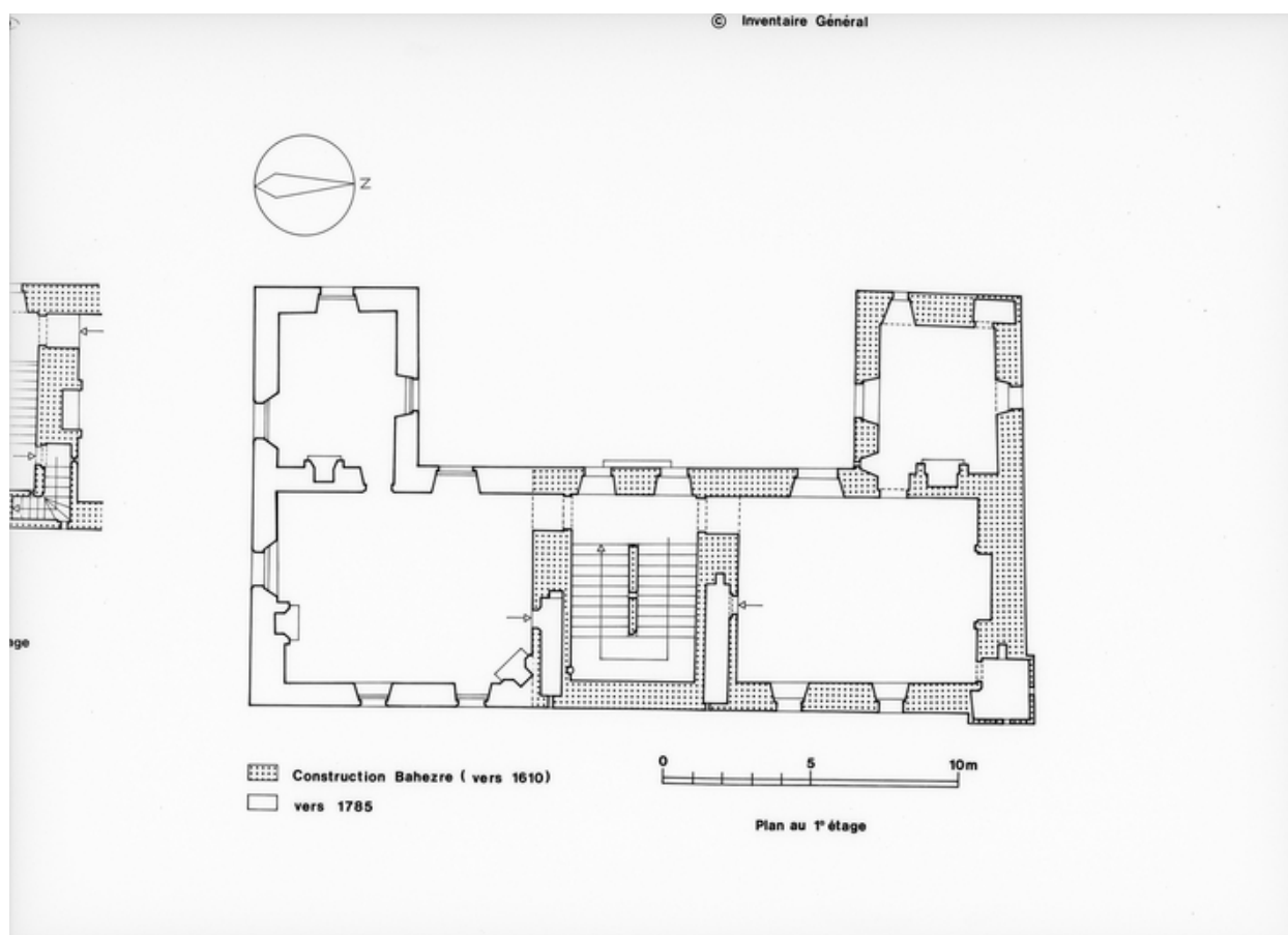
Plan : 1er étage (plan archéologique)
