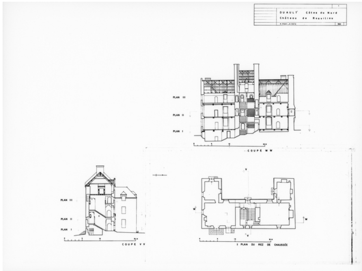
Plan et coupes
