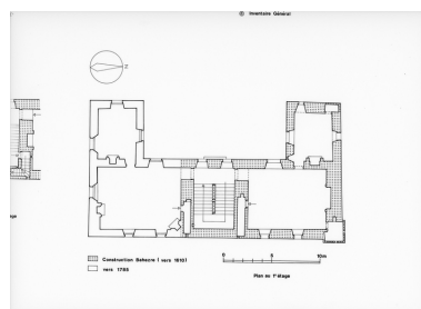
Plan : 1er étage (plan archéologique) Phot. Guy Artur, Phot. Norbert Lambart IVR53_19892200002P
