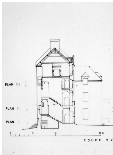
Coupe V-V Phot. Guy Artur, Autr. P Boutroux IVR53_19762200376P
