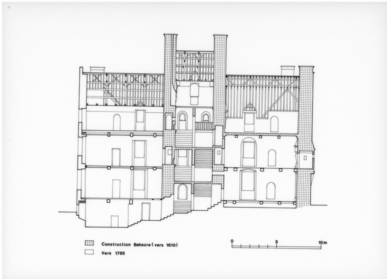
Coupe avec époques de construction
