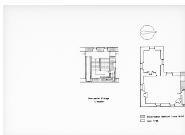
Plan partiel, 2ème étage : l'escalier Phot. Guy Artur, Phot. Norbert Lambart IVR53_19892200001P
