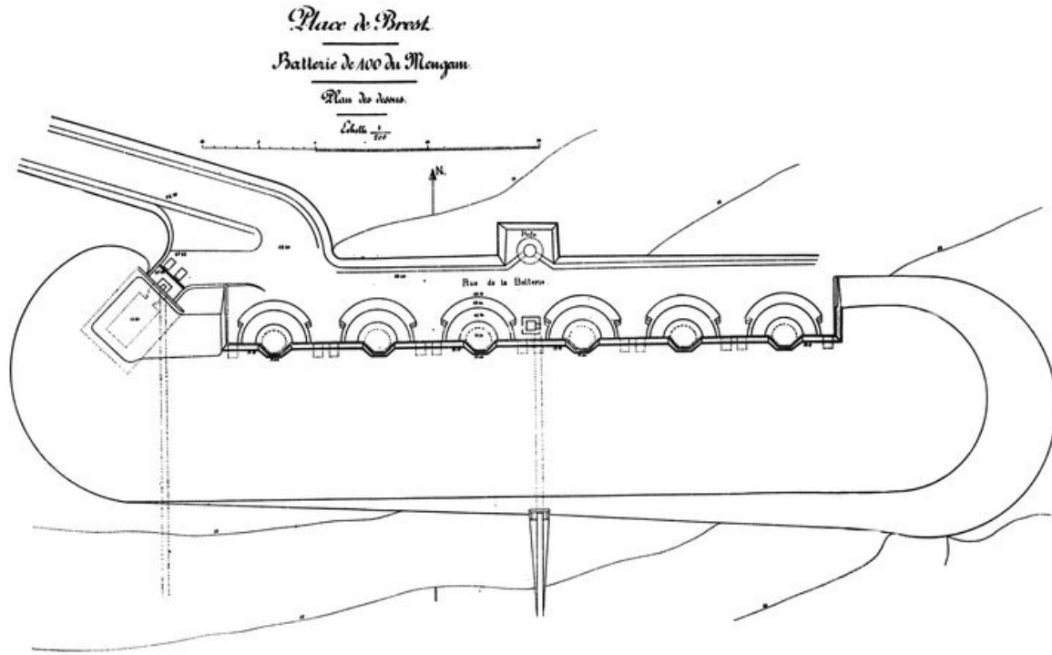
Plan de la batterie extérieure de 100 mm du Mengant, Atlas des batteries de côte : côte de Brest, fin 19e siècle
