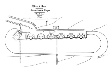
Plan de la batterie extérieure de 100 mm du Mengant, Atlas des batteries de côte : côte de Brest, fin 19e siècle Phot. Guy Artur, Phot. Norbert Lambart, Autr. IVR53_19702900052Z
