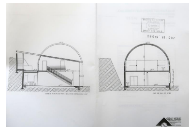
Ateliers et salles de technologie, coupes. Gildas Nédélec, architecte, 26 mars 1993. Autr. Gildas Nédélec IVR53_20212905058A3
