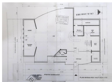
Centre de documentation et d'information : plan du rez-de-chaussée haut. Gildas Nédélec, architecte, 1er juin 1995. Autr. Gildas Nédélec IVR53_20212905060A3
