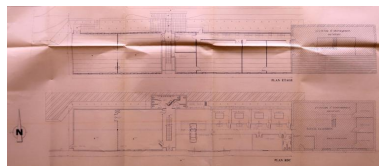
Ateliers et salles de technologie, plans rez-de-chaussée et étage. Gildas Nédélec, architecte, 26 mars 1993. Autr. Gildas Nédélec IVR53_20212905057A0
