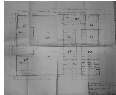
Construction d'un atelier de matériaux composites haute performance. René Le Friant, architecte, 27/11/1987. Autr. René Le Friant IVR53_20212905049A1
