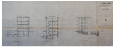
Bâtiment N, externat : façade sud et coupes AA, BB, façade est. J-B. Mathon, architecte, sd. Autr. Jean-Baptiste Mathon IVR53_20212905048A0
