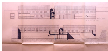
Ateliers et salles de technologie, façades sud et nord. Gildas Nédélec, architecte, 26 mars 1993. Autr. Gildas Nédélec IVR53_20212905056A0
