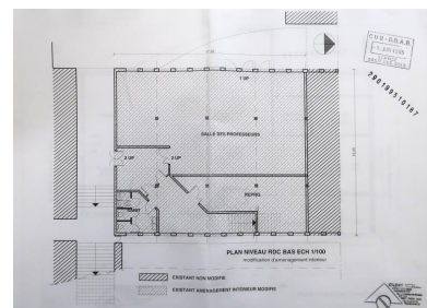
Centre de documentation et d'information : plan du rez-de-chaussée bas. Gildas Nédélec, architecte, 1er juin 1995. Autr. Gildas Nédélec IVR53_20212905059A3
