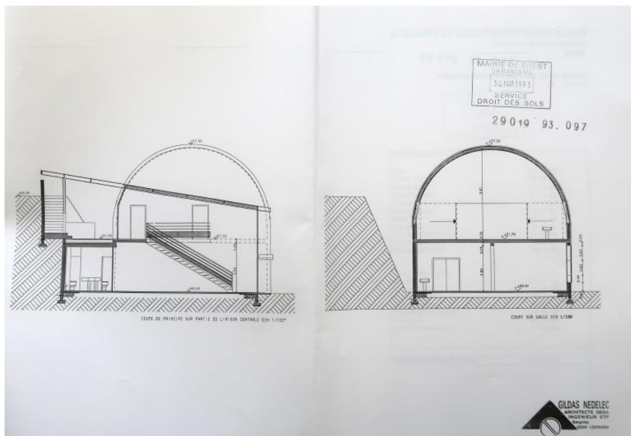
Ateliers et salles de technologie, coupes. Gildas Nédelec, architecte, 26 mars 1993.
