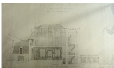
Projet Phot. Norbert Lambart IVR53_20063501424NUCA
