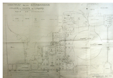
Projet Phot. Norbert Lambart IVR53_20063501423NUCA
