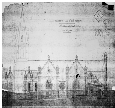
Élévation latérale Sud n°4. Phot. Guy Artur, Phot. Norbert Lambart, Autr. Arthur Regnault IVR53_19973500155X
