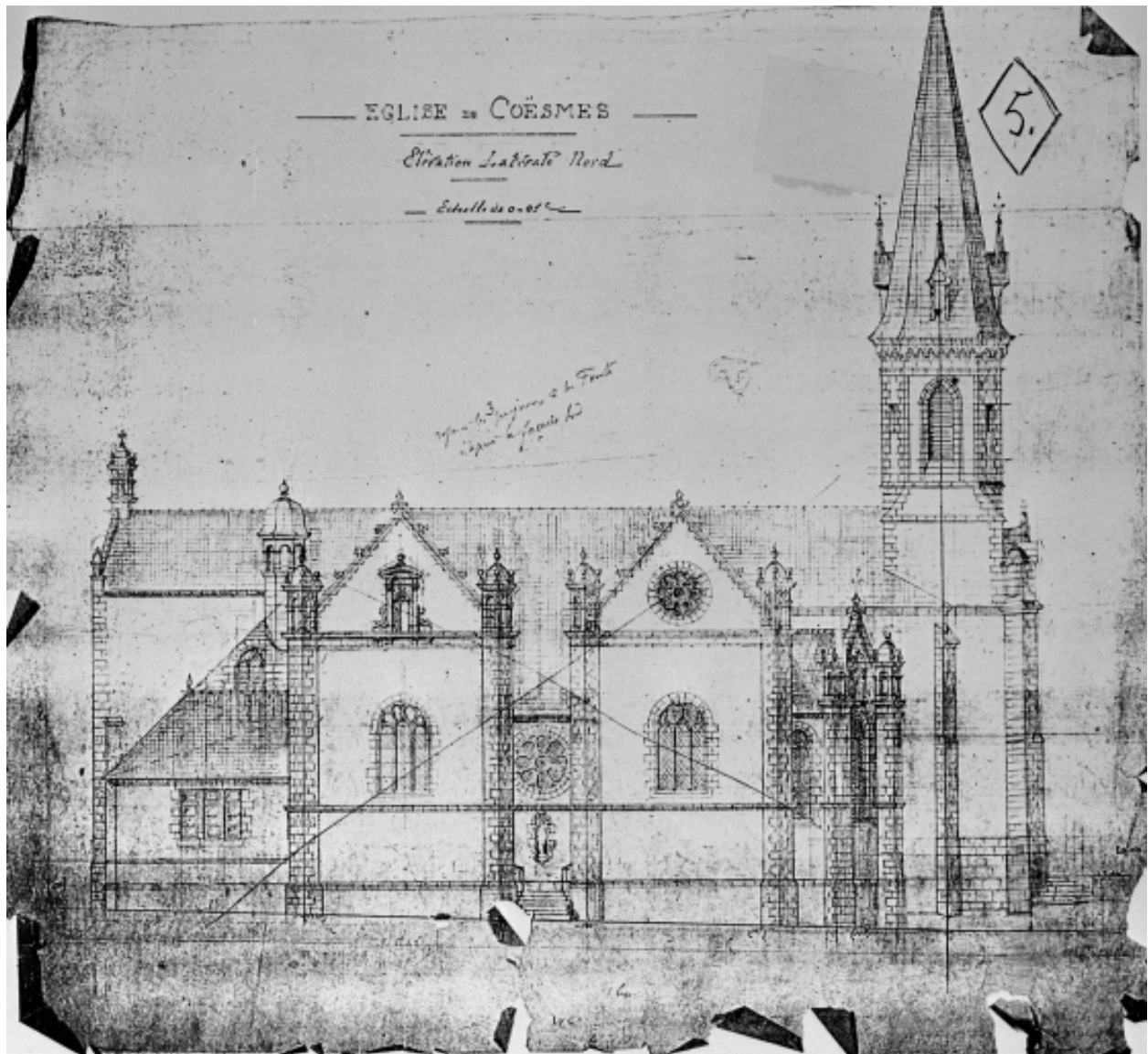
Élévation latérale Nord n°5.
