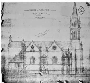
Élévation latérale Nord n°5. Phot. Guy Artur, Phot. Norbert Lambart, Autr. Arthur Regnault IVR53_19973500156X
