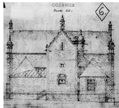
Élévation de la façade Est n°6. Phot. Guy Artur, Phot. Norbert Lambart, Autr. Arthur Regnault IVR53_19973500234X
