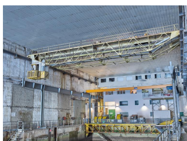
Vue du fond de l'alvéole depuis le quai (bassin abritant les emplacements 21 et 22). Les anciens ateliers sont en cours de réhabilitation. Au premier plan, pont roulant d'origine et au second plan, pont roulant récent avec son chemin de roulement Phot. Bernard Bègne IVR53_20235600577NUCA
