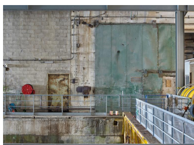
Vue de la porte coulissante située entre les alvéoles B et C avec son système d'ouverture par treuil. Elle est également dotée d'une porte piétonne. Sur la porte, on peut lire : NEFS CLIMATISEES REFERMEZ CETTE PORTE APRES VOTRE PASSAGE Phot. Bernard Bègne IVR53_20235600580NUCA
