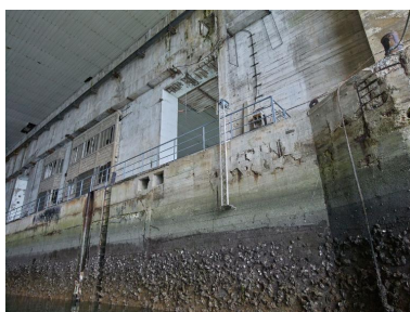
Vue de l'alvéole C (n ° 21 et 22) : quai est Phot. Bernard Bègne IVR53_20215600506NUCA
