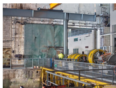
Vue de la porte coulissante située entre les alvéoles B et C avec son système d'ouverture par treuil. Elle est également dotée d'une porte piétonne. Sur la porte, on peut lire : NEFS CLIMATISEES REFERMEZ CETTE PORTE APRES VOTRE PASSAGE Phot. Bernard Bègne IVR53_20235600579NUCA
