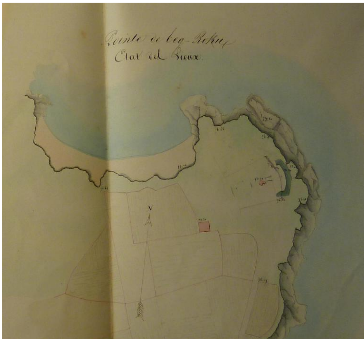
1 VH 1518. Place de Quiberon, feuille des projets pour 1847, batteries de Beg Rohu et de Beg Quilvi, 12 avril 1847.
