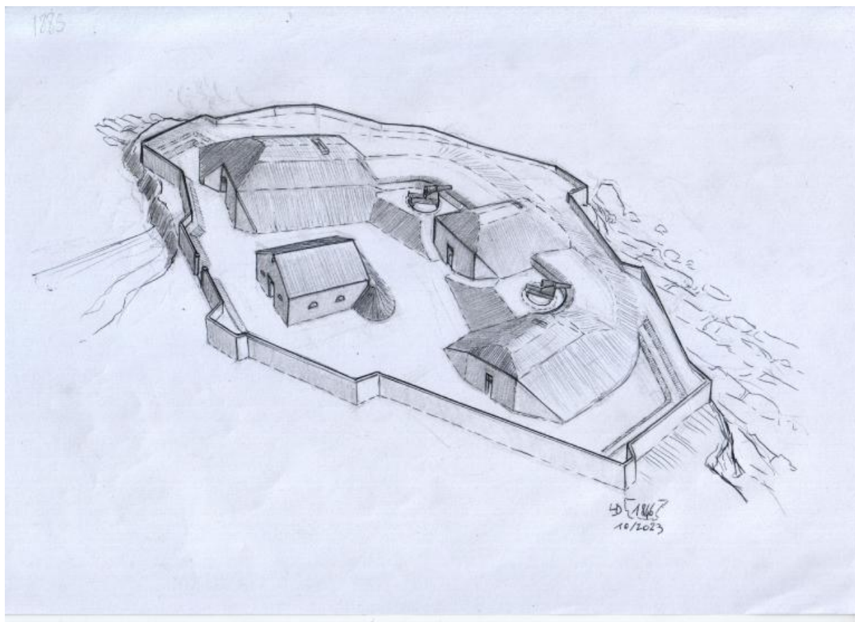
Saint-Pierre-Quiberon, Batterie de Beg Rohu, évocation de l'état vers 1890, par Lionel Duigou.
