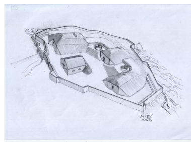
Saint-Pierre-Quiberon, Batterie de Beg Rohu, évocation de l'état vers 1890, par Lionel Duigou. Autr. Lionel Duigou IVR53_20235605354NUCA
