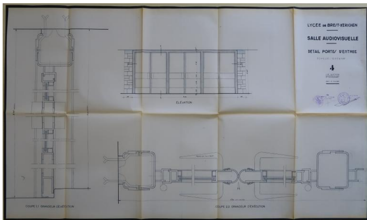
Salle audiovisuelle. Détail portes d'entrée. Jean-Baptiste Mathon, architecte, 5 février 1963.
