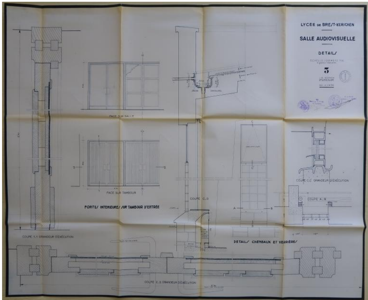
Salle audiovisuelle. Détails. Jean-Baptiste Mathon, architecte, 5 février 1963.
