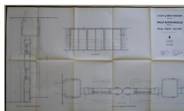
Salle audiovisuelle. Détail portes d'entrée. Jean-Baptiste Mathon, architecte, 5 février 1963. Autr. Jean-Baptiste Mathon IVR53_20222905016A0
