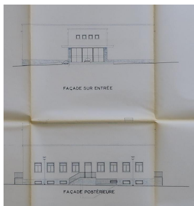
Salle audiovisuelle. Façades sur entrée et postérieure. Jean-Baptiste Mathon, architecte, 5 février 1963. Autr. Jean-Baptiste Mathon IVR53_20222905014A0
