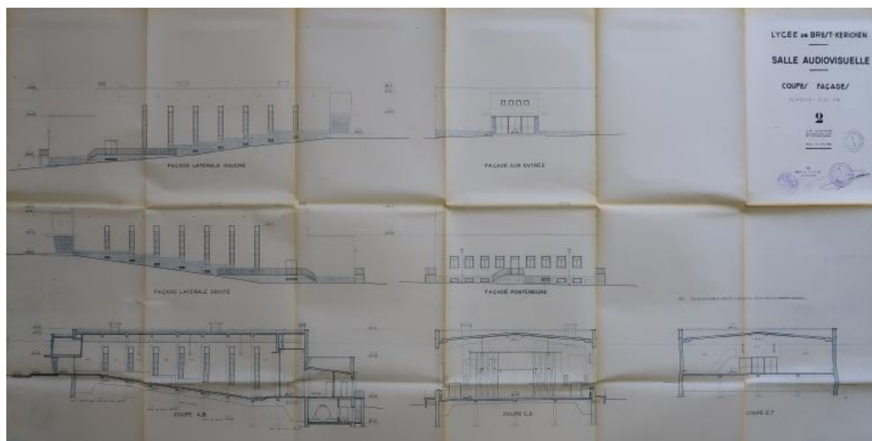
Salle audiovisuelle. Coupes - façades. Jean-Baptiste Mathon, architecte, 5 février 1963.
