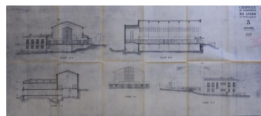
Chapelle et aumônerie du lycée. Coupes. Jean-Baptiste Mathon, architecte, 28.5.58. Autr. Jean-Baptiste Mathon IVR53_20222905206A0
