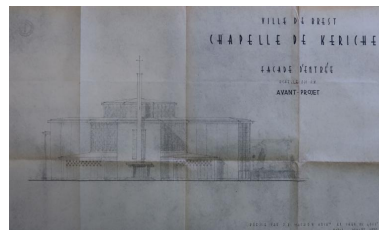
Chapelle de Kerichen, façade d'entrée. Avant-Projet. Jean-Baptiste Mathon, architecte, Juillet 1952. Autr. Jean-Baptiste Mathon IVR53_20222905004A0
