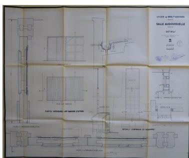
Salle audiovisuelle. Détails. Jean-Baptiste Mathon, architecte, 5 février 1963. Autr. Jean-Baptiste Mathon IVR53_20222905015A0
