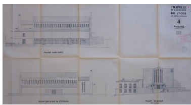
Chapelle et aumônerie du lycée. Façades. Jean-Baptiste Mathon, architecte, 28.5.58. Autr. Jean-Baptiste Mathon IVR53_20222905007A0
