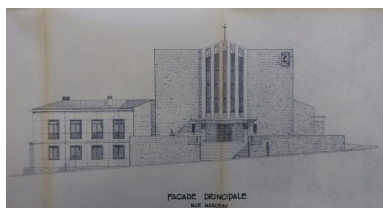
Chapelle et aumônerie du lycée. Façade principale, rue Marceau. Jean-Baptiste Mathon, architecte, 28.5.58. Autr. Jean-Baptiste Mathon IVR53_20222905008A0
