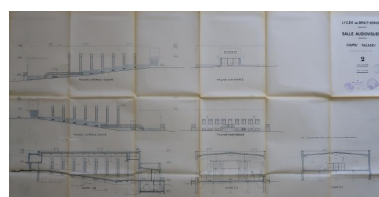
Salle audiovisuelle. Coupes - façades. Jean-Baptiste Mathon, architecte, 5 février 1963. Autr. Jean-Baptiste Mathon IVR53_20222905013A0
