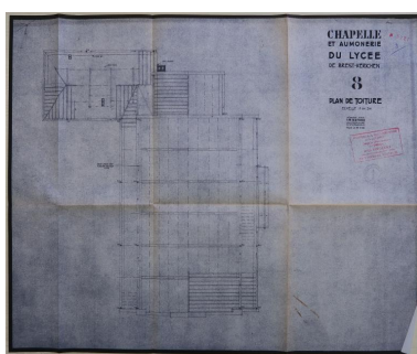
Chapelle et aumônerie du lycée. Plan de toiture. Jean-Baptiste Mathon, architecte, 28.5.58. Autr. Jean-Baptiste Mathon IVR53_20222905009A0
