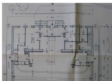
Salle audiovisuelle. Détail des aménagements côté scène. Jean-Baptiste Mathon, architecte, 5 février 1963. Noter les rails qui permettent d'amener l'autel sur le devant de la scène, afin de dire les messes et la présence de deux aumôneries, pour les garçons et pour les filles, pour la pratique religieuse en semaine. Autr. Jean-Baptiste Mathon IVR53_20222905207A0
