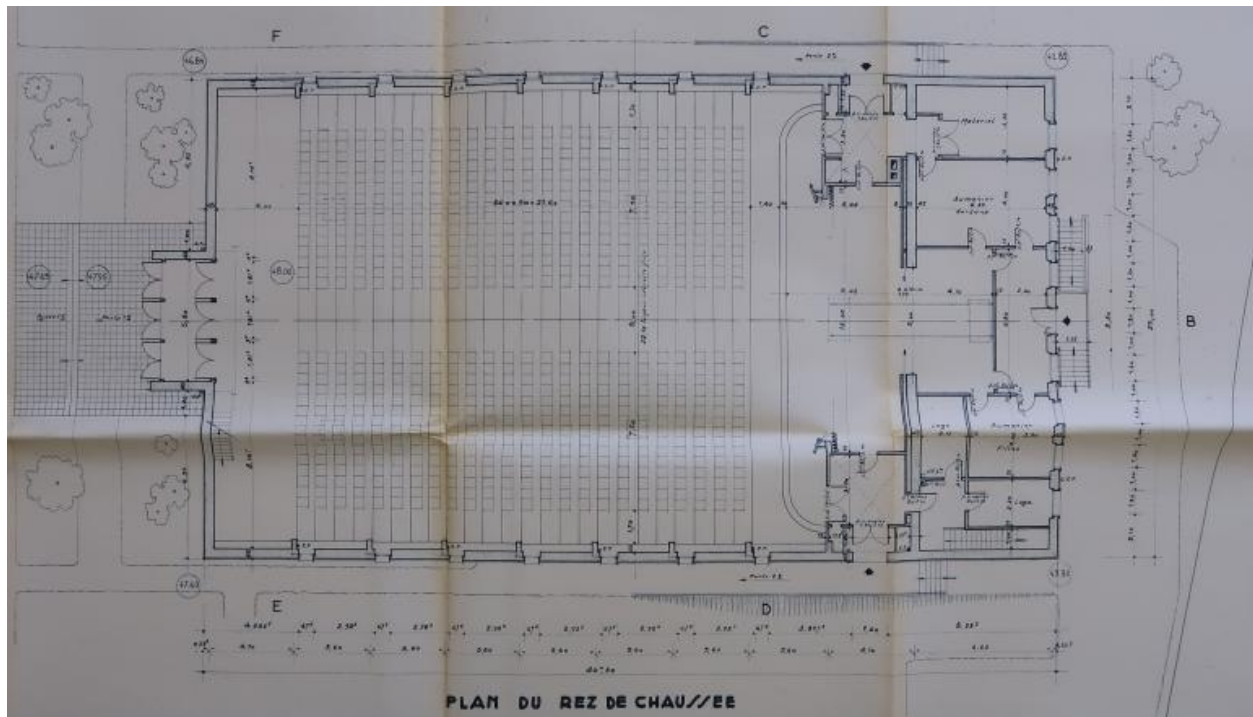
Salle audiovisuelle. Plan du rez-de-chaussée. Jean-Baptiste Mathon, architecte, 5 février 1963.
