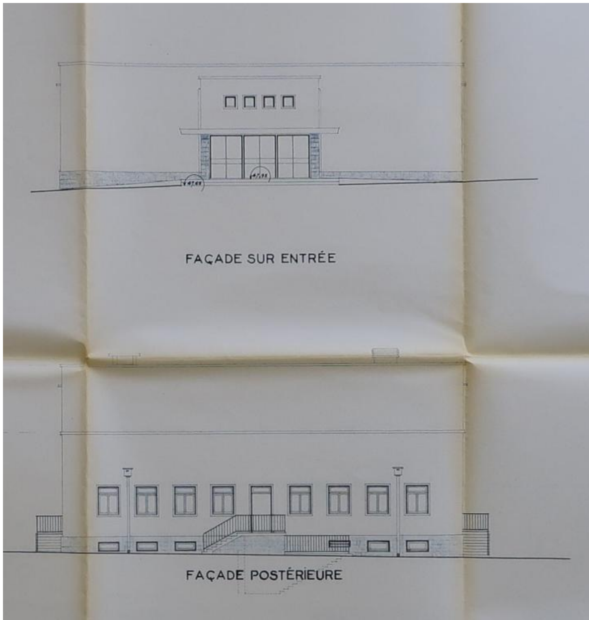
Salle audiovisuelle. Façades sur entrée et postérieure. Jean-Baptiste Mathon, architecte, 5 février 1963.
