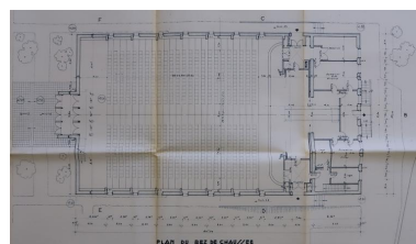
Salle audiovisuelle. Plan du rez-de-chaussée. Jean-Baptiste Mathon, architecte, 5 février 1963. Autr. Jean-Baptiste Mathon IVR53_20222905012A0
