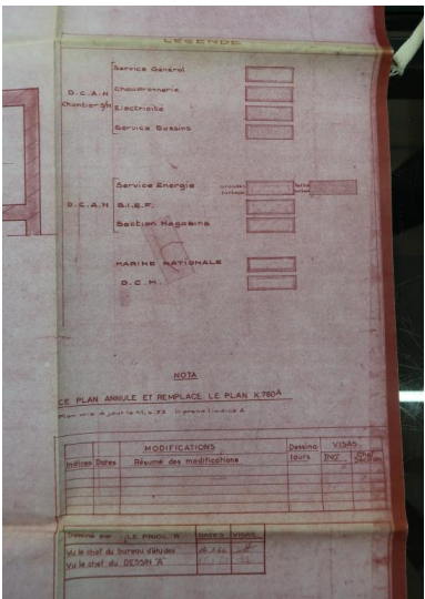
Extrait du plan du bloc n° 1, distribution des locaux : cartouche, plan K n° 780A, 28 décembre 1965,
