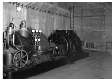
Vue du groupe turbo-dynamo situé au premier étage de l'extension sud : extrémité est avec débouché de l'escalier, photographie non datée (collection : Archives municipales de Lorient) Phot. Anonyme IVR53_20235605334NUCA
