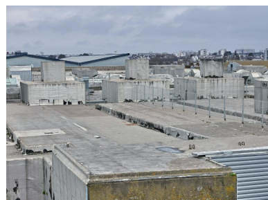
Vue de situation des trois cheminées de la chaudferie depuis la dalle de couverture du bunker KI. Au premier plan, dalle supérieure de l'accès des trémies à charbon
