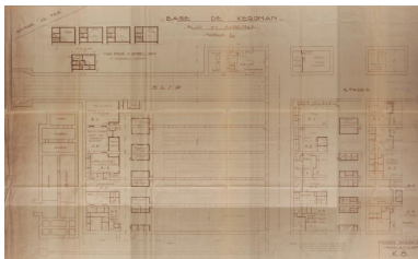
Plan d'ensemble du bunker KI, plan K n° 8, 10 novembre 1945 (Service Historique de la Défense de Lorient, Monographie de la base "Ingénieur Général Stosskopf", 1945-1946) Phot. Service Historique de la Défense IVR53_20235605301NUCA
