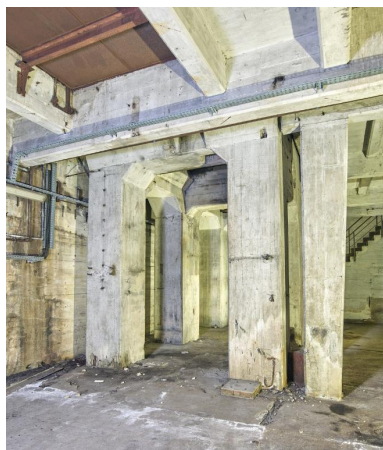
Vue de la salle du condenseur (fonction en 1945) puis atelier (fonction en 1966) dans l'extension sud : piliers en béton armé supportant le plafond sur lequel est implanté un groupe turbo-dynamo (mentionné en 1945). En arrière-plan : l'escalier d'accès au premier étage Phot. Bernard Bègne IVR53_20235600165NUCA
