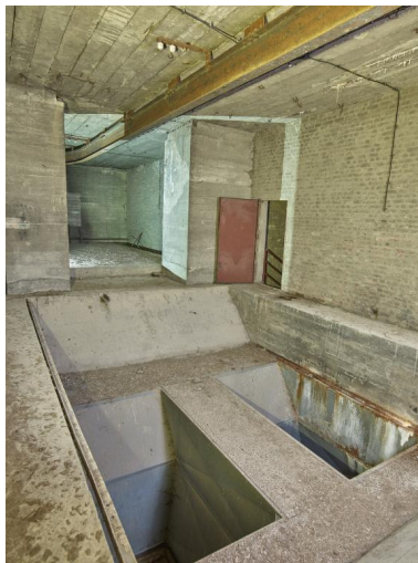
Vue du deuxième étage de l'extension sud : couloir d'accès aux trémies à charbon, monorail avec son système d'alimentation électrique triphasée. Au premier plan, l'une des trois trémies
