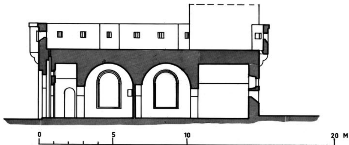
COUPE V-V
