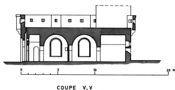
COUPE V.V
