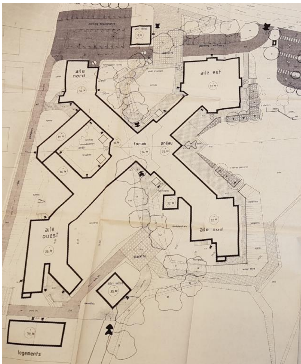
Plan masse. Espaces verts. Voirie nivellement : détail sur les bâtiments. Patrick Pincemaille, architecte, 1986.
