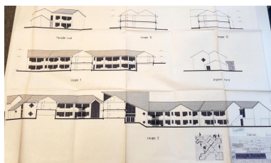
Coupe. façades. Patrick Pincemaille architecte, 1986. Dess. Patrick Pincemaille IVR53_20185606514A0
