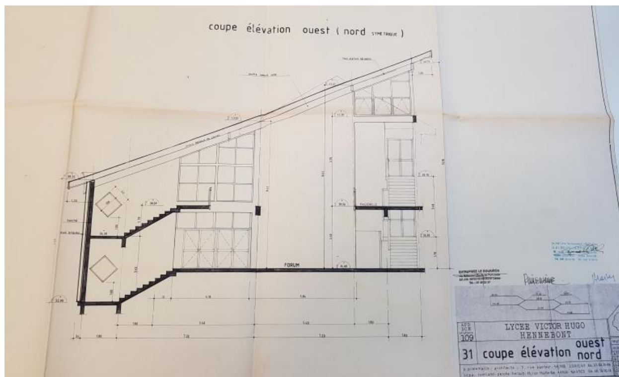
Coupe élévation ouest nord.
