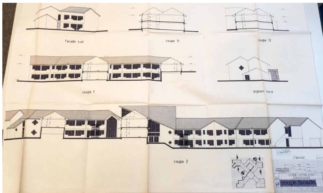
Coupe. façades. Patricik Pincemaille architecte, 1986.
