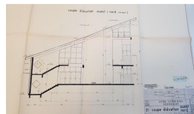
Coupe élévation ouest nord. Dess. Patrick Pincemaille IVR53_20185606515A0
