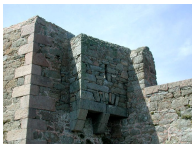
Vue de la bretèche flanquant le pont-levis de la redoute, réduit de l'île aux Moines Phot. Guillaume Lécueillier
