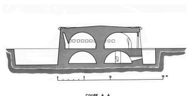
Coupe A-A du réduit de la pointe des Espagnols Repro. Guy Artur, Repro. Norbert Lambert, Phot. Auteur inconnu, Autr. Coignat Autret IVR53_19872900213P
