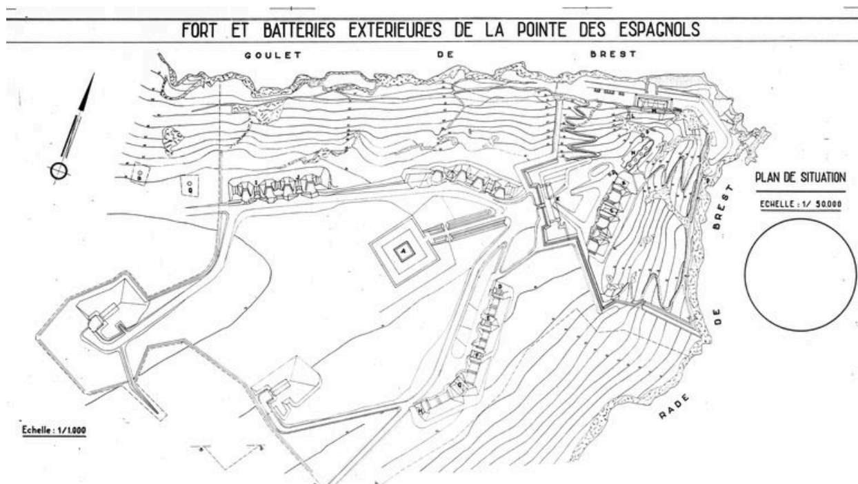
Plan d'ensemble du fort et batteries de la pointe des Espagnols
