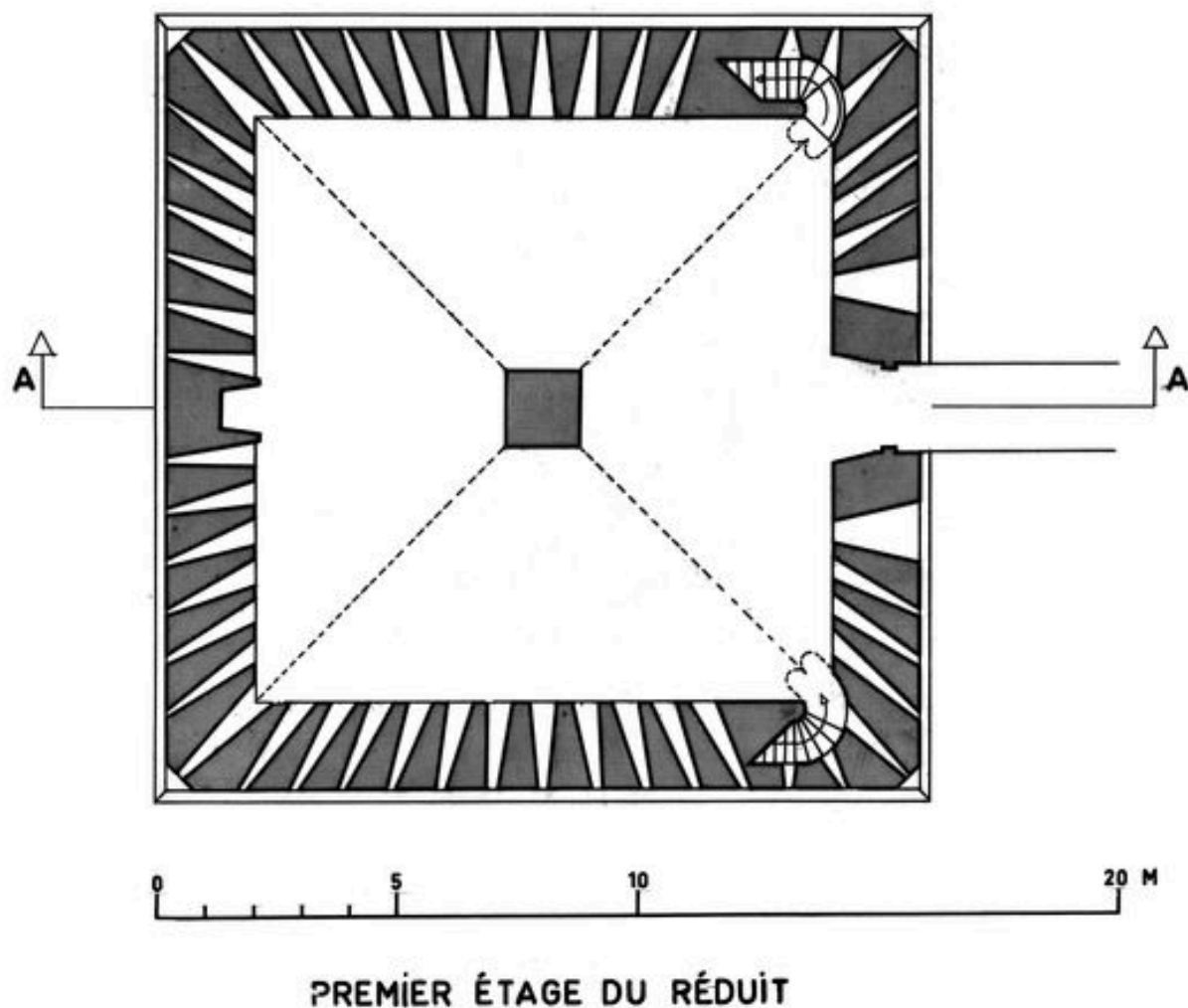
Plan du premier étage du réduit de la pointe des Espagnols
