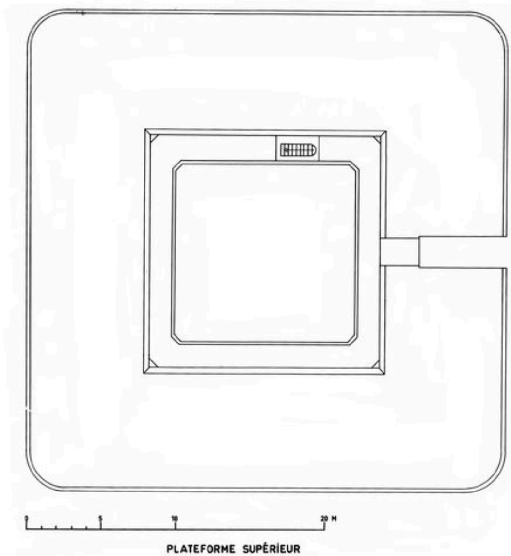
Plan du réduit de la pointe des Espagnols avec son fossé sec
