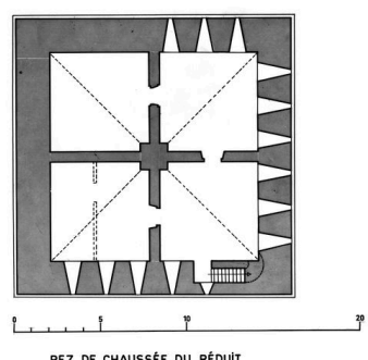
Plan du rez-de-chaussée du réduit de la pointe des Espagnols Repro. Guy Artur, Repro. Norbert Lambert, Phot. Auteur inconnu, Autr. Coignat Autret IVR53_19872900211P
