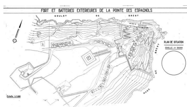
Plan d'ensemble du fort et batteries de la pointe des Espagnols Repro. Guy Artur, Repro. Norbert Lambert, Phot. Auteur inconnu, Autr. Coignat Autret IVR53_19872900158P
