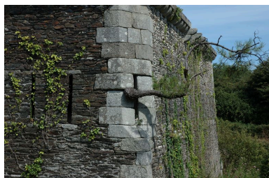
Vue de la tour-modèle n° 1 type 1811 de la pointe des Espagnols Phot. Guillaume Lécueillier IVR53_20072906410NUCA
