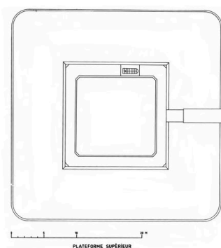
Plan du réduit de la pointe des Espagnols avec son fossé sec Repro. Guy Artur, Repro. Norbert Lambert, Phot. Auteur inconnu, Autr. Coignat Autret IVR53_19872900210P
