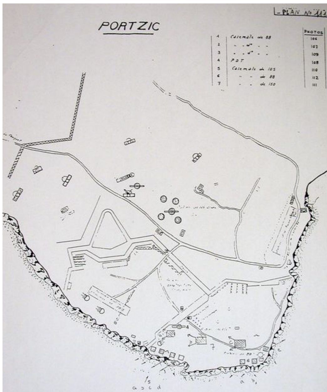
Plan de l'ensemble fortifié du Portzic, n° 111, rapport Pinczon du Sel. Livre IV, vers 1947, Service Historique de la Marine, Brest
