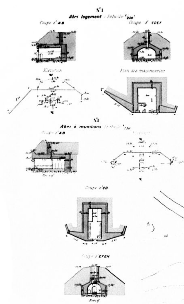
Plan et coupes de l'abri logement n° 1 et de l'abri à munitions de la batterie Nationale du fort de mer du Portzic (2 canons M de 32 cm modèle 1870-1881), Direction d'Artillerie du génie de Brest, 1893, par le colonel Directeur d'Artillerie : Collomb Repro. Guillaume Lécullier IVR53_20052904182NUC
