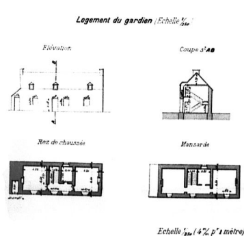
Plan et coupes du logement du gardien de la batterie du fort de mer, Direction d'Artillerie du génie de Brest, 1893 Repro. Guillaume Lécueillier IVR53_20052904179NUC
