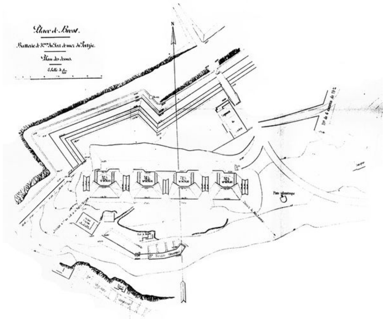
Plan de la batterie du fort de mer (4 canons de 32 cm modèle 1870-1881)
