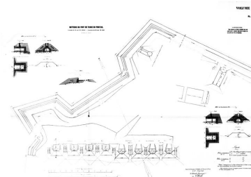
Plan de la batterie du fort de terre du Portzic (Batterie de 32 cm et batterie de mortiers de 30 cm), Direction d'Artillerie du génie de Brest, 1893 Repro. Guy Artur, Repro. Norbert Lambart IVR53_19702900082Z
