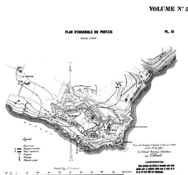
Plan d'ensemble du Portzic, Direction d'Artillerie du génie de Brest, 1893 Repro. Guy Artur, Repro. Norbert Lambart IVR53_19702900081Z
