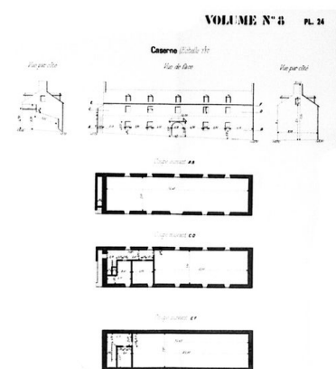
Plan et coupes de la caserne du fort de mer, Direction d'Artillerie du génie de Brest, 1893 Repro. Guillaume Lécueillier IVR53_20052904181NUC
