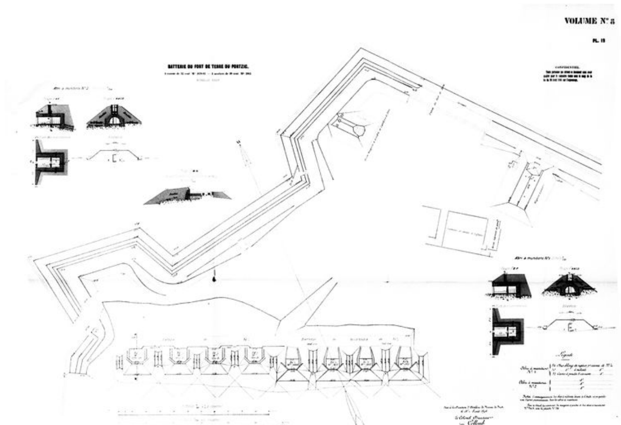
Plan de la batterie du fort de terre du Portzic (Batterie de 32 cm et batterie de mortiers de 30 cm), Direction d'Artillerie du génie de Brest, 1893
