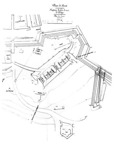
Plan de la batterie du fort de mer (4 canons de 19 cm modèle 1864-1866) Repro. Guy Artur, Repro. Norbert Lambart IVR53_19702900060Z
