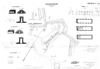
Plan et coupes de la batterie du fort de mer (4 canons de 19 cm), Direction d'Artillerie du génie de Brest, 1893 Repro. Guy Artur, Repro. Norbert Lambart IVR53_19702900087Z
