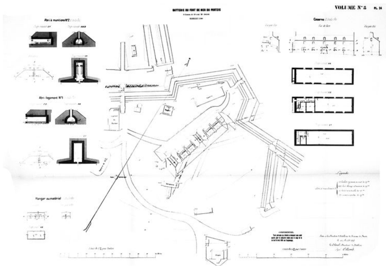
Plan et coupes de la batterie du fort de mer (4 canons de 19 cm), Direction d'Artillerie du génie de Brest, 1893
