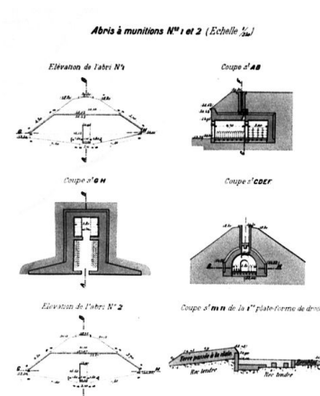
Plan et coupes des abris à munitions n° 1 et 2 de la batterie du fort de mer, Direction d'Artillerie du génie de Brest, 1893 Repro. Guillaume Lécueillier IVR53_20052904180NUC
