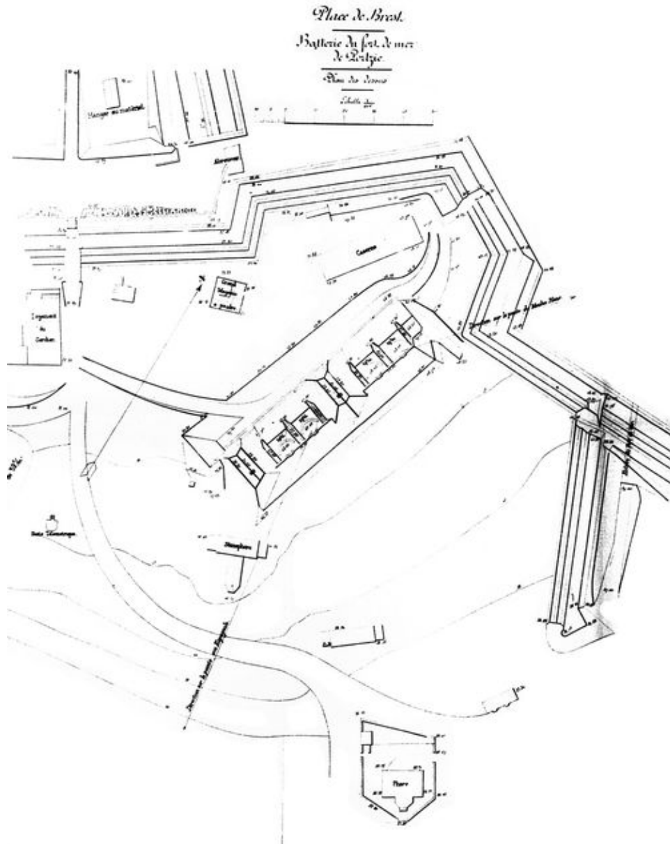
Plan de la batterie du fort de mer (4 canons de 19 cm modèle 1864-1866)
