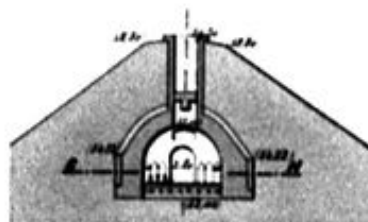
Coupe s' mn de la 1 re plate-forme de droite
