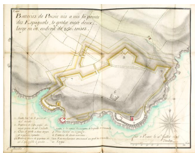
Plan des batteries du Portzic, fait à Brest le 15 juillet 1695 et signé par Vauban (Collection : Bibliothèque du Génie) Repro. Service Historique de la Défense, Autr. Sébastien Le Prestre de Vauban IVR53_20082908815NUCA
