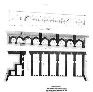
Plan et coupes des casemates du fort du de terre du Portzic, Direction d'Artillerie du génie de Brest, 1893 Repro. Guillaume Lécullier IVR53_20052904177NUC
