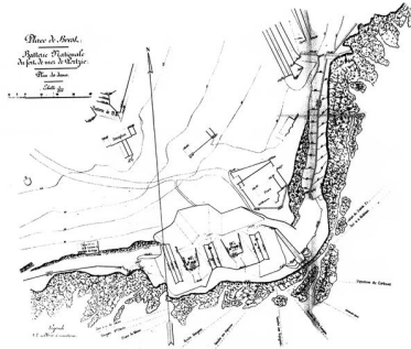
Plan de la batterie Nationale du fort de mer du Portzic (2 canons de 32 cm modèle 1870-1881)
