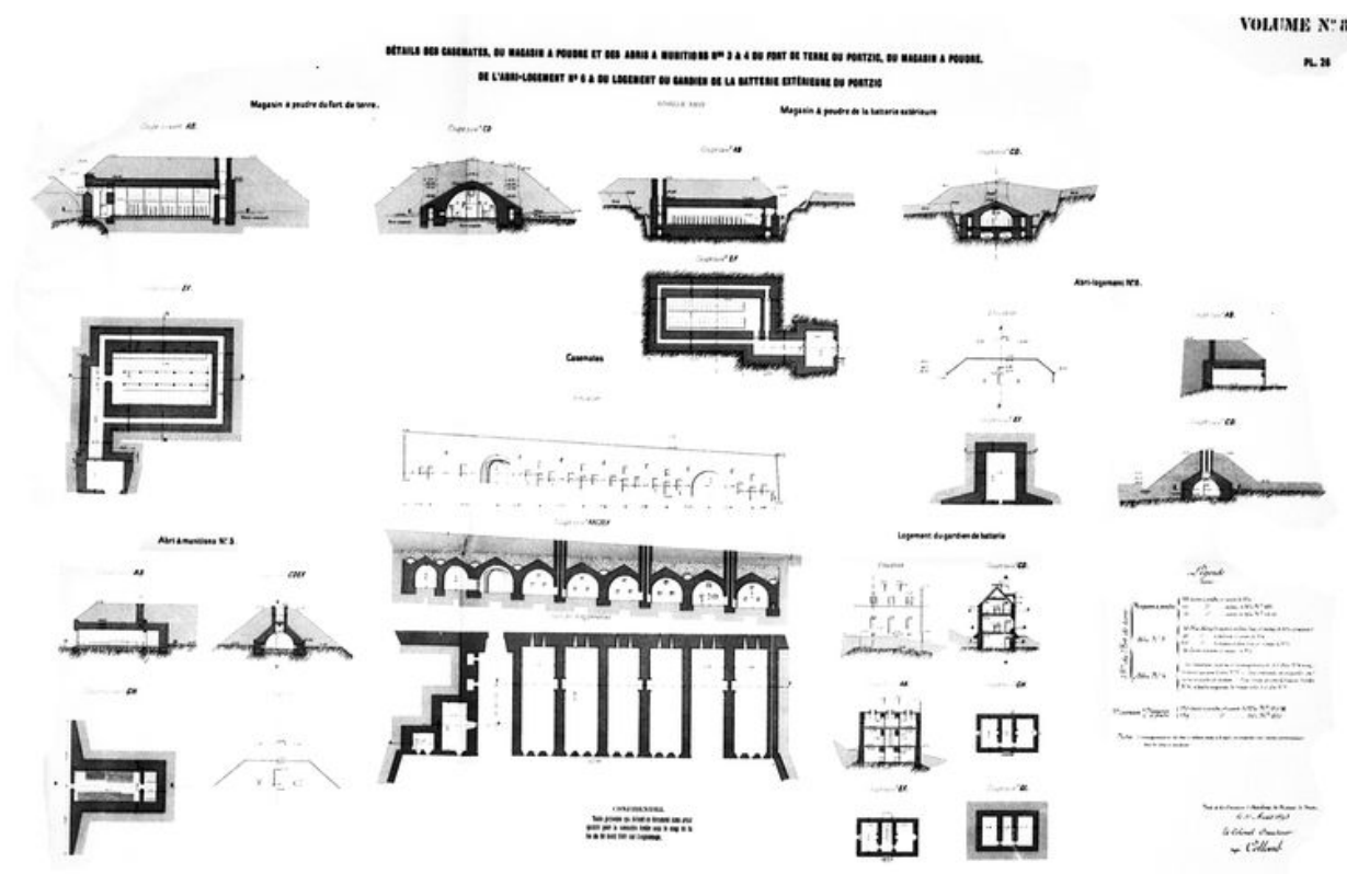
Détail des casernes, du magasin à poudre et des abris à munitions n° 3 et 4 du fort de terre du Portzic, du magasin à poudre, de l'abri-logement n° 6 et du logement du gardien, Direction d'Artillerie du génie de Brest, 1893
