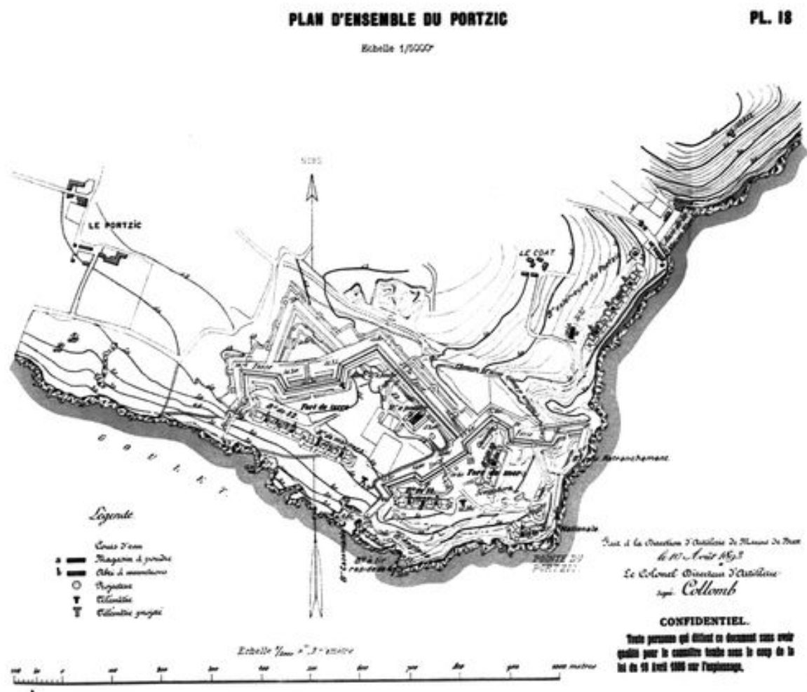
Plan d'ensemble du Portzic, Direction d'Artillerie du génie de Brest, 1893
