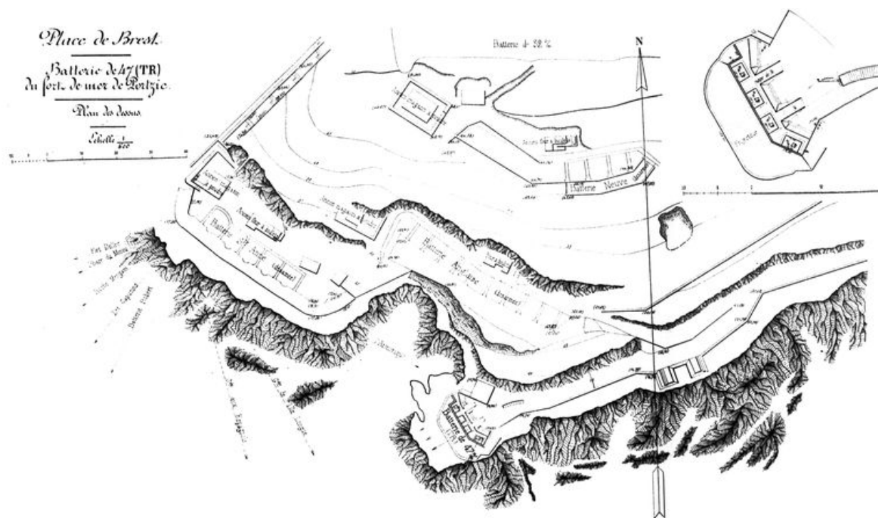
Plan de la batterie à tir rapide du fort de mer du Portzic (4 canons de 47 mm modèle 1885)
