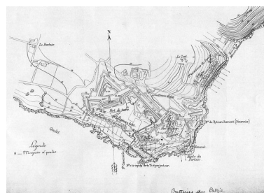
Plan d'ensemble du Portzic, 1913 (Atlas des batteries de côte) Repro. Guillaume Lécullier IVR53_20032901763NUC
