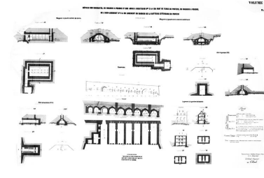
Détail des casemates, du magasin à poudre et des abris à munitions n° 3 et 4 du fort de terre du Portzic, du magasin à poudre, de l'abri-logement n° 6 et du logement du gardien, Direction d'Artillerie du génie de Brest, 1893 Repro. Guy Artur, Repro. Norbert Lambart IVR53_19702900089Z
