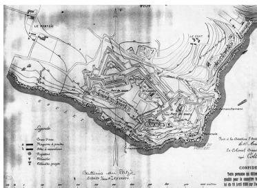
Plan du fort du Portzic, 1893 Repro. Guillaume Lécueillier IVR53_20032901762NUC
