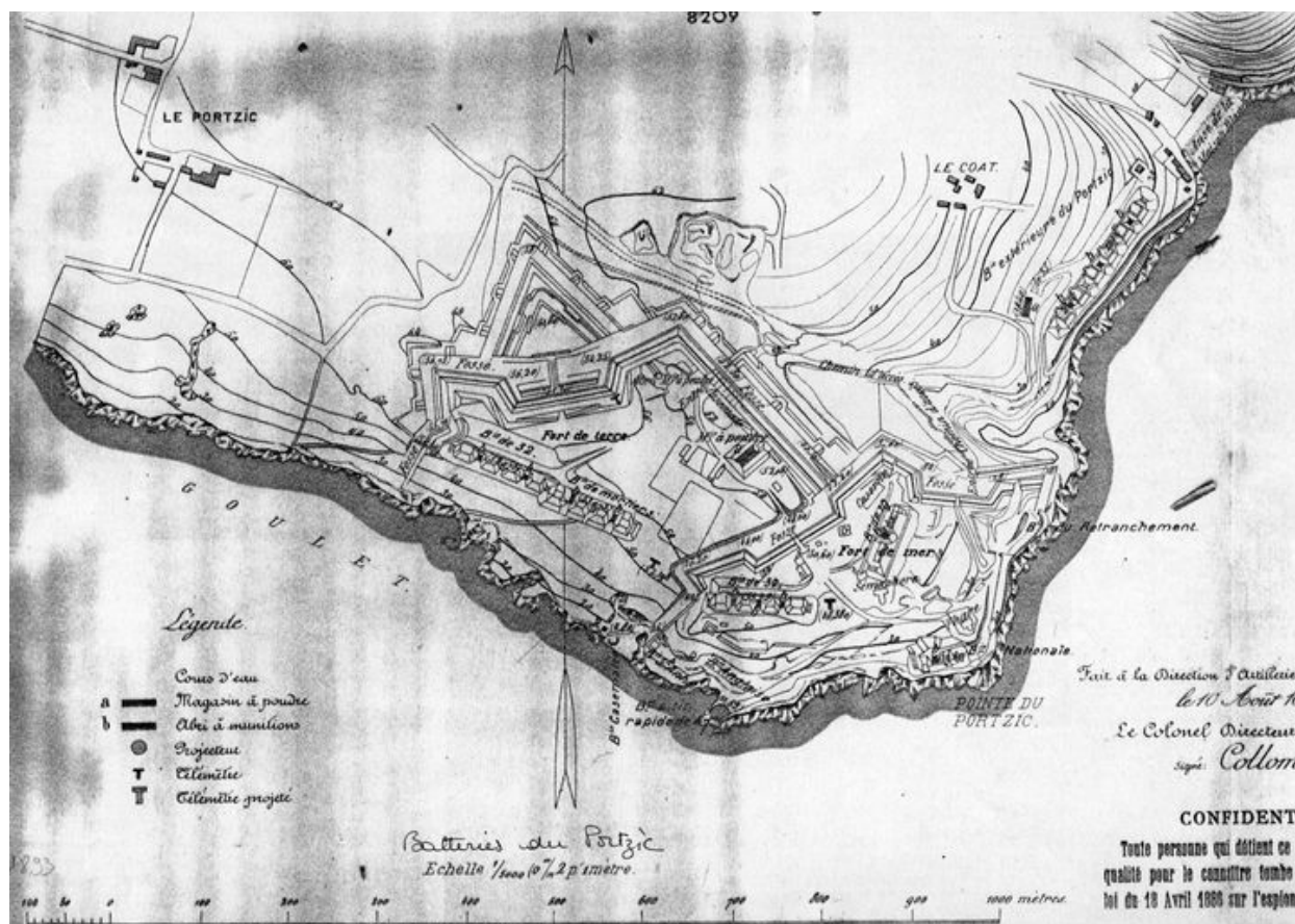
Plan du fort du Portzic, 1893
