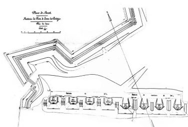
Plan de la batterie du fort de terre du Portzic (Batterie de 32 cm et batterie de mortiers de 30 cm) Repro. Guy Artur, Repro. Norbert Lambart IVR53_19702900056Z
