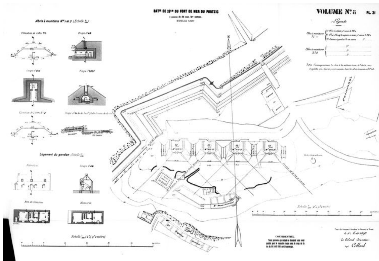
Plan et coupes de la batterie du fort de mer (4 canons de 32 cm modèle 1870-1881), Direction d'Artillerie du génie de Brest, 1893
