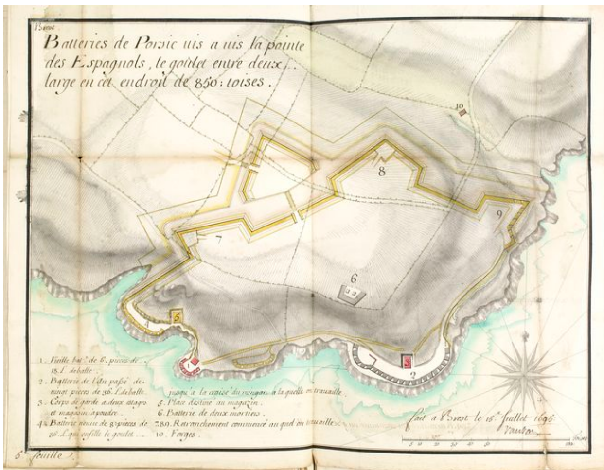
Plan des batteries du Portzic, fait à Brest le 15 juillet 1695 et signé par Vauban (Collection : Bibliothèque du Génie)
