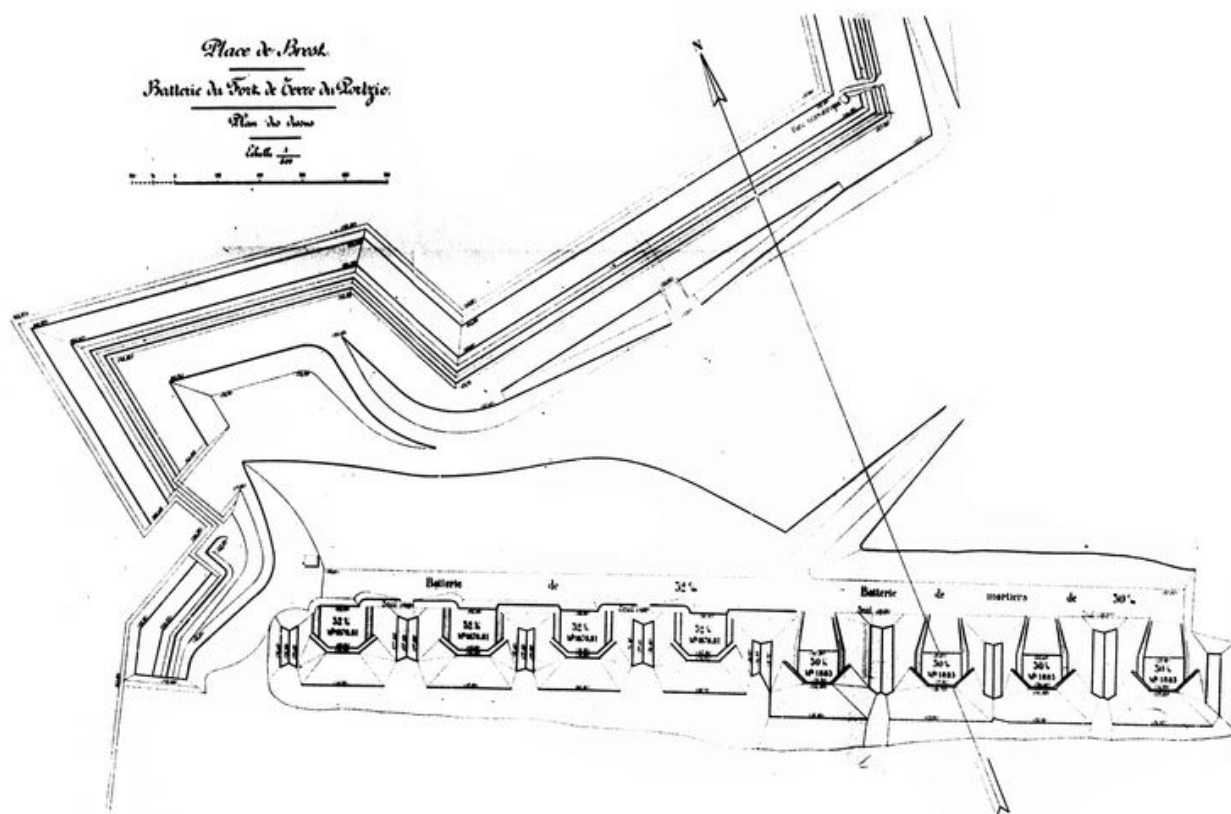
Plan de la batterie du fort de terre du Portzic (Batterie de 32 cm et batterie de mortiers de 30 cm)
