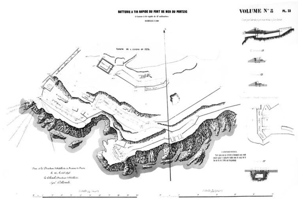
Plan et coupes de la batterie à tir rapide du fort de mer du Portzic (4 canons de 47 mm modèle 1885), Direction d'Artillerie du génie de Brest, 1893
