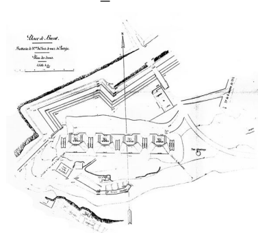
Plan de la batterie du fort de mer (4 canons de 32 cm modèle 1870-1881) Repro. Guy Artur, Repro. Norbert Lambart IVR53_19702900058Z
