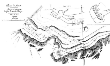
Plan de la batterie à tir rapide du fort de mer du Portzic (4 canons de 47 mm modèle 1885)
