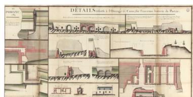
Détail relatif à l'ouvrage à corne sur l'ancienne batterie du Portzic (plans, coupes et élévations), 1784 (Collection : Archives départementales du Finistère) Phot. Archives départementales du Finistère IVR53_20222905406NUCA
