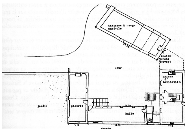
Plan au sol de la maison et de ses dépendances (CAUE 22, Bernard Belorgey, 1998) Phot. Bernard Belorgey IVR53_20222206018NUCA
