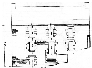
Relevé de la façade antérieure de la maison (CAUE 22, Bernard Belorgey, 1998) Phot. Bernard Belorgey IVR53_20222206015NUCA
