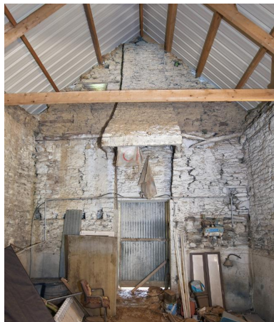
Remise nord-ouest. Pignon nord. Vue intérieure avec les traces des différents niveaux : cheminée de l'étage en surcroît, emplacements des embouts de poutres du plancher, sablière du plafond. Phot. Bernard Bègne IVR53_20232200175NUCA
