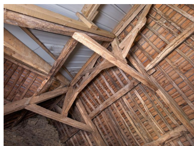
Logis sur dépendance construit en retour d'équerre de la sècherie. Charpente à sous-faîtage avec croix-de-Saint-André et liens pour affermer les angles par triangulation. Phot. Bernard Bègne IVR53_20232200186NUCA
