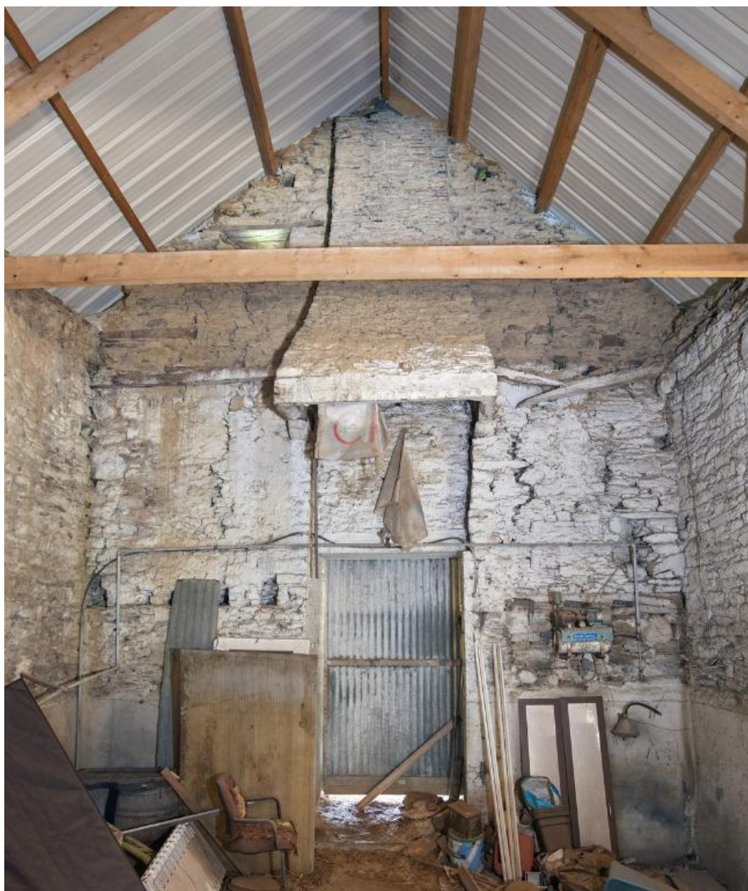
Remise nord-ouest. Pignon nord. Vue intérieure avec les traces des différents niveaux : cheminée de l'étage en surcroît, emplacements des embouts de poutres du plancher, sablière du plafond.
