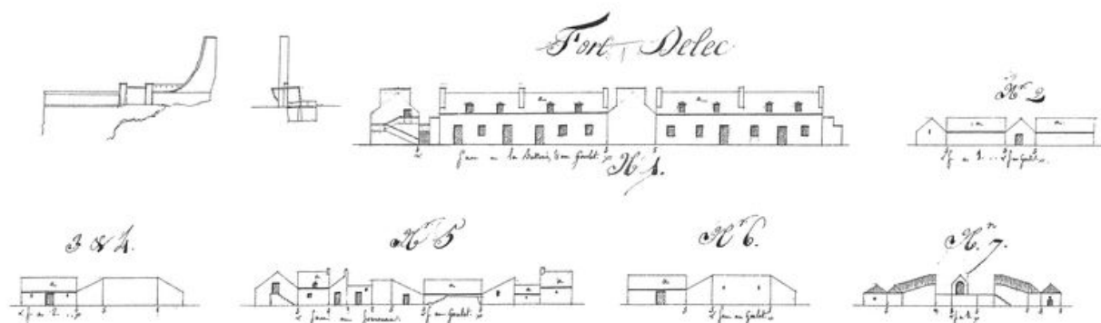
Développements des forts du camp retranché et des batteries de la côte du nord, année 1807. Fort du Dellec [Dellec]. Divers bâtiments, n° 1 à 7. Fourneau à rougir les boulets
