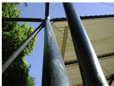
Vue du fort du Dellec : structure légère et toile assurant l'étanchéité de l'espace de la caserne aujourd'hui réhabilité Phot. Guillaume Lécueillier IVR53_20052903412NUCA
