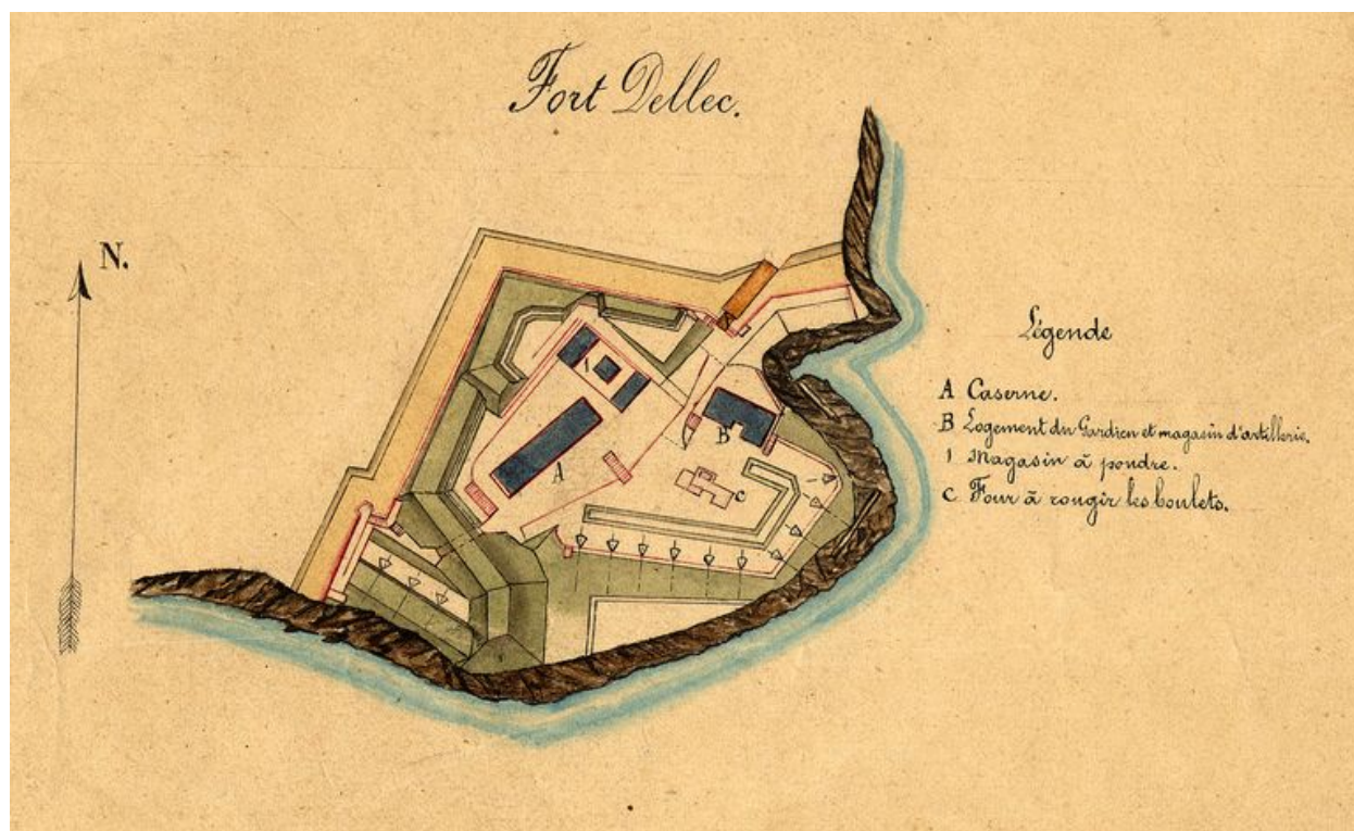
Plan du fort du Dellec : batteries, caserne, logement du gardien, magasin d'artillerie, magasin à poudre et four à rougir les boulets, Génie, Direction de Brest, 1ère moitié 19e siècle
