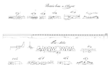
Développements des forts du camp retranché et des batteries de la côte du nord, année 1807. Batterie basse du Mingant [Mengant]. Divers bâtiments, n° 9 à 13. Fourneau à rougir les boulets. Fort du Delec [Dellec]. Divers bâtiments, n° 1 à 7 Repro. Christian Carlet, Repro. Guillaume Lécueillier, Autr. Boitard aîné IVR53_20062907177NUCA
