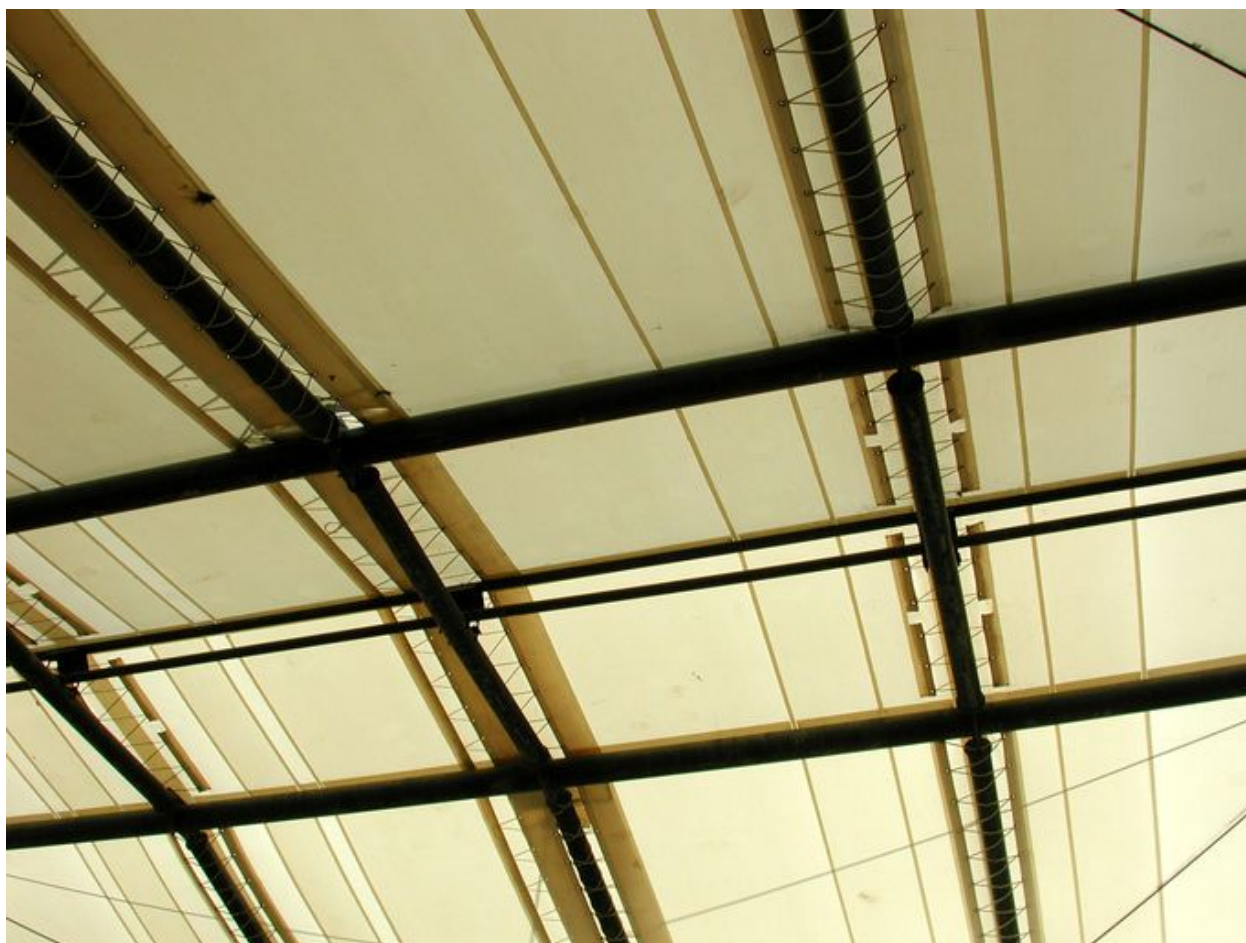
Vue du fort du Dellec : structure légère et toile assurant l'étanchéité de l'espace de la caserne aujourd'hui réhabilité
