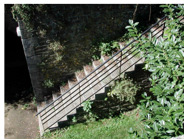
Vue du fort du Dellec : escalier permetant l'accès à la plate- forme et au parapet de l'escarpe Phot. Guillaume Lécueillier IVR53_20052903417NUCA
