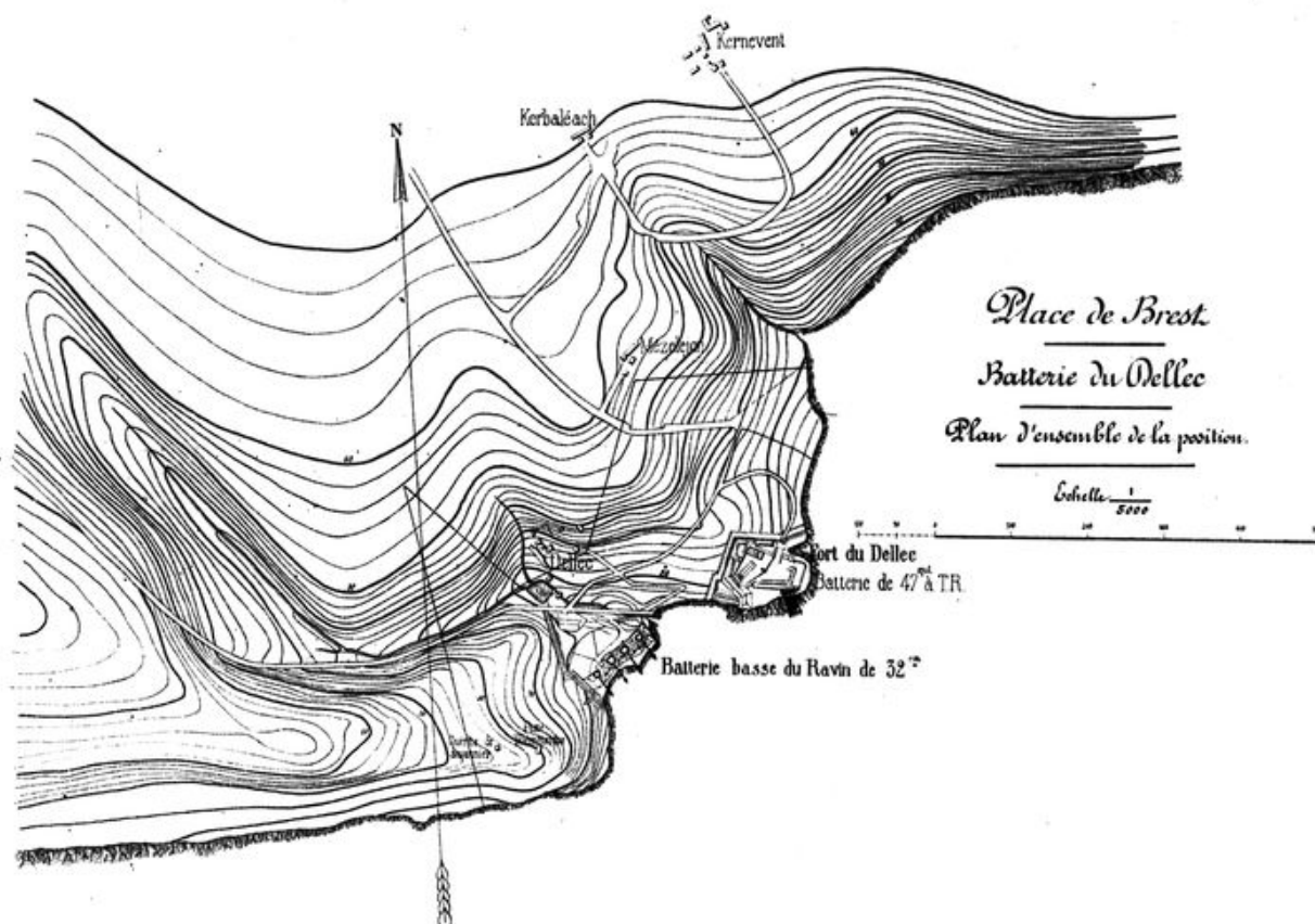
Plan de situation des batteries de Dellec
