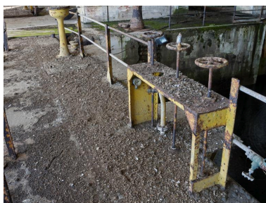
Vue des commandes des vannes de ballast du bateau-porte fermant le bassin (vers l'intérieur) Phot. Bernard Bègne IVR53_20235600634NUCA
