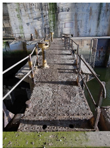
Vue des commandes des pompes et vannes du bateau- porte fermant le bassin Phot. Bernard Bègne IVR53_20235600632NUCA
