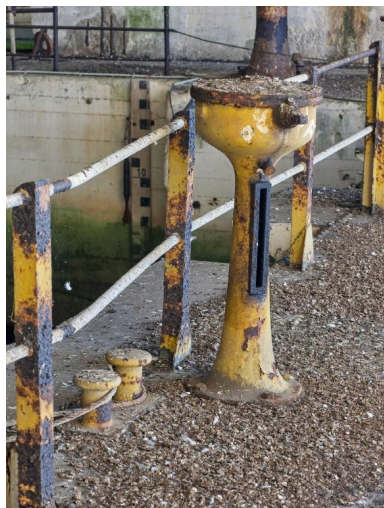
Vue de l'une des deux commandes de pompe sur le bateau-porte fermant le bassin. Elle fonctionnait avec une manivelle Phot. Bernard Bègne IVR53_20235600636NUCA
