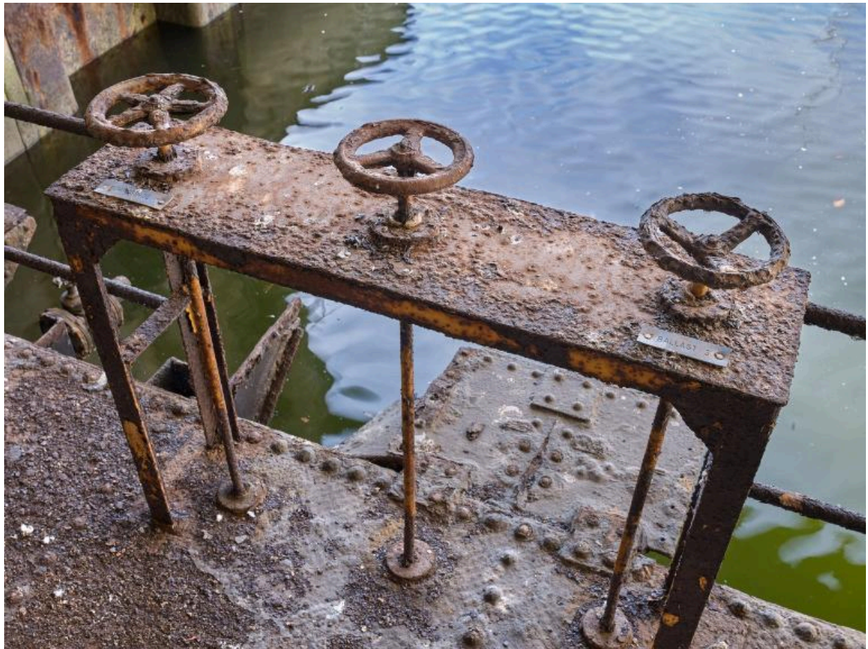
Vue des commandes des vannes du bateau-porte fermant le bassin (vers l'extérieur). On peut lire de gauche à droite : REPLISSAGE 1, [plaque disparue, 2], BALLAST 3
