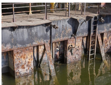
Vue de détail du bateau-porte fermant le bassin : prises d'air pour le remplissage du ballast ? Phot. Bernard Bègne IVR53_20235600631NUCA
