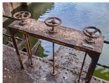
Vue des commandes des vannes du bateau-porte fermant le bassin (vers l'extérieur). On peut lire de gauche à droite : REMPLISSAGE 1, [plaque disparue, 2], BALLAST 3 Phot. Bernard Bègne IVR53_20235600635NUCA
