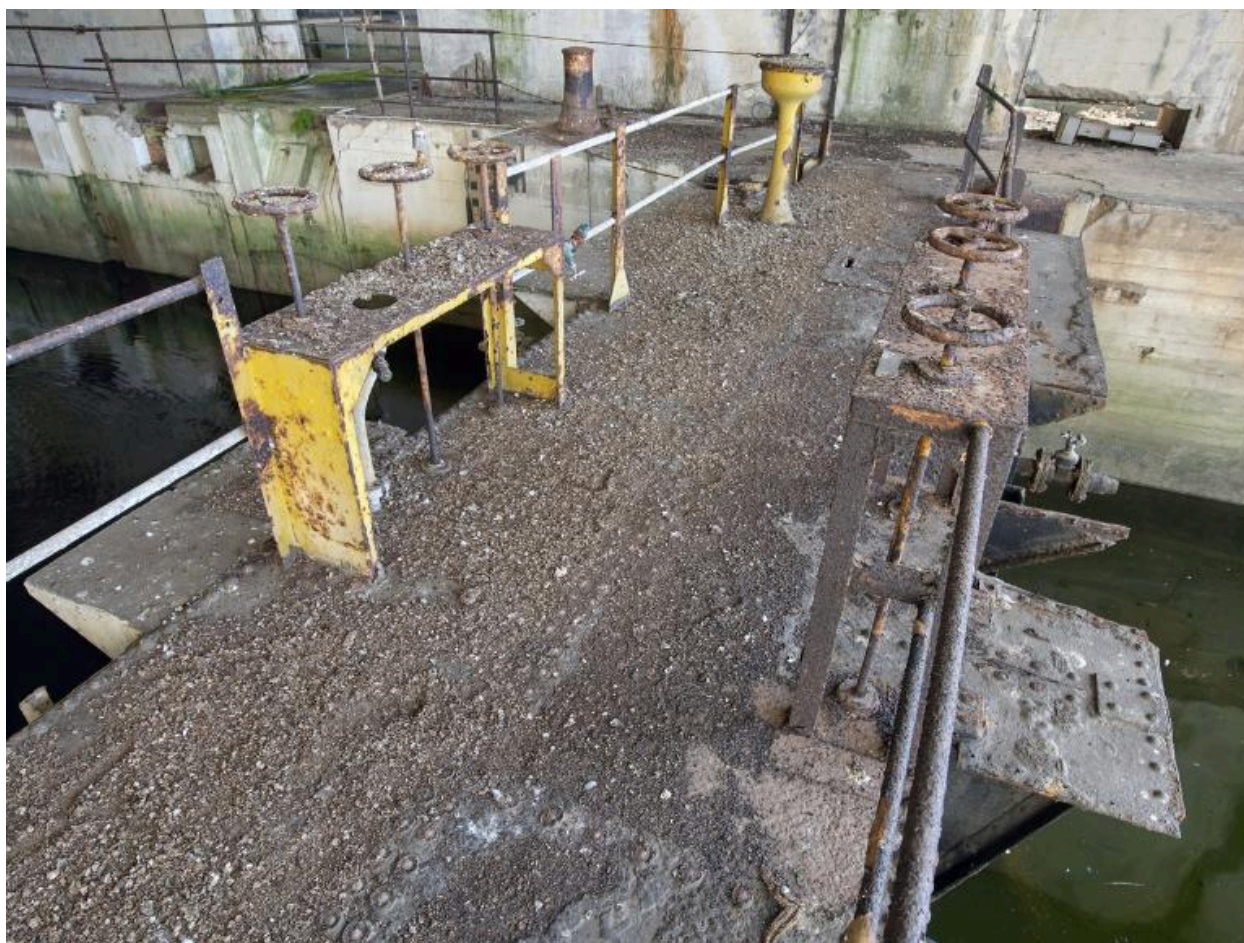
Vue des commandes des vannes du bateau-porte fermant le bassin (vers l'intérieur et vers l'extérieur)
