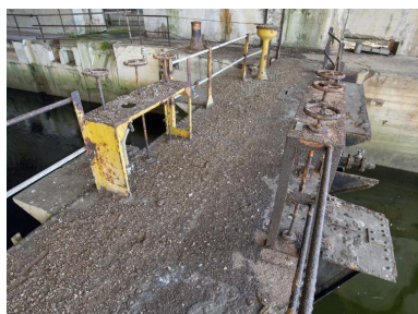
Vue des commandes des vannes du bateau-porte fermant le bassin (vers l'intérieur et vers l'extérieur) Phot. Bernard Bègne IVR53_20235600633NUCA
