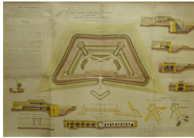
1 VK 141. Étude d'une batterie fermée rédigée en 1847 par Mr le général du génie Noizet. Phot. Patrick Jadé IVR53_20172906489NUCA
