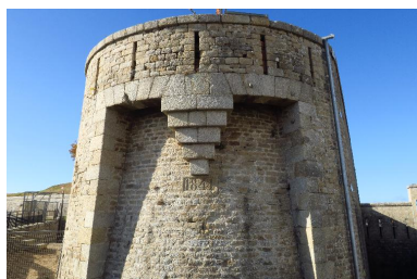
Saint-Pierre-Quiberon, fort de Penthievre, créneaux de pied et parapet crénelé. Phot. Lionel Duigou IVR53_20175606653NUCA
