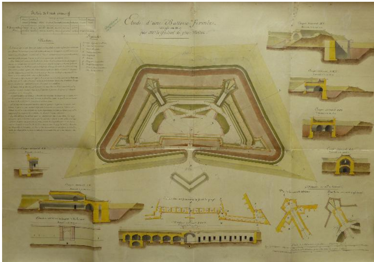
1 VK 141. Étude d'une batterie fermée rédigée en 1847 par Mr le général du génie Noizet.
