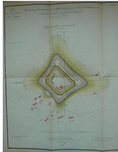
1 VH 657. Place du Conquet, feuille n° 9 des projets supplémentaires pour 1858-1859, construire le réduit central de l'île d'Ouessant, 18 décembre 1858.
