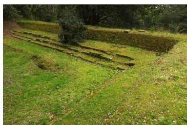
Le Palais, enceinte urbaine, courtine 21-22, parapet d'infanterie avec banquette en maçonnerie. Phot. Lionel Duigou IVR53_20175608431NUCA
