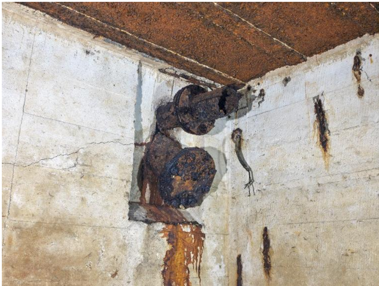
Vue de détail de l'extrémité ouest de la salle de garde : conduit de cheminée (en haut) et conduit de ramonage (en bas) du poêle. Dans le mur, passage de câble électrique du magasin à munitions
