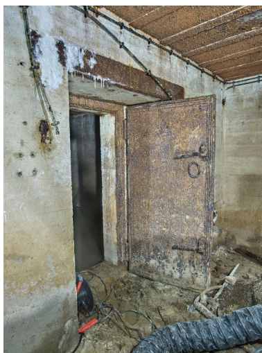
Vue de détail de la porte blindée étanche du magasin
