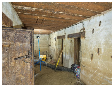
Vue de la salle de garde avec ses deux portes étanches d'accès. Au premier plan à gauche, la porte étanche du magasin à munitions ouest. Phot. Bernard Bègne IVR53_20253501365NUCA
